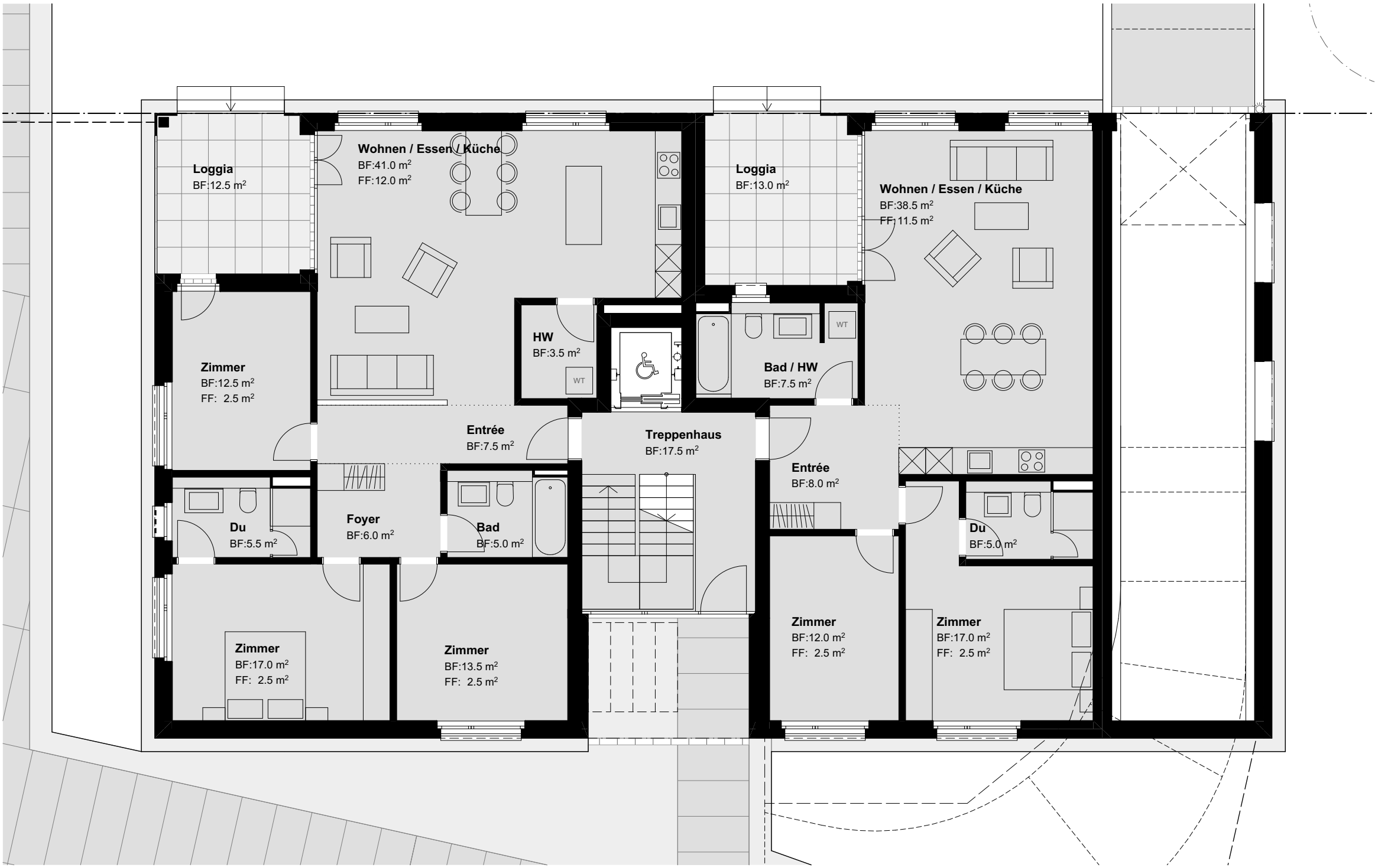
Haus A, Grundriss Erdgeschoss
