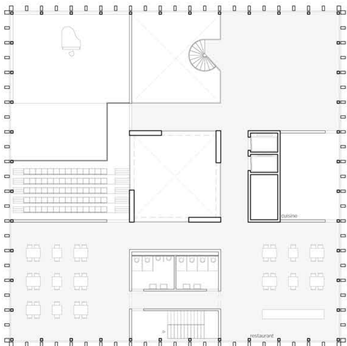
7ème étage salles d'auditions_1:200
