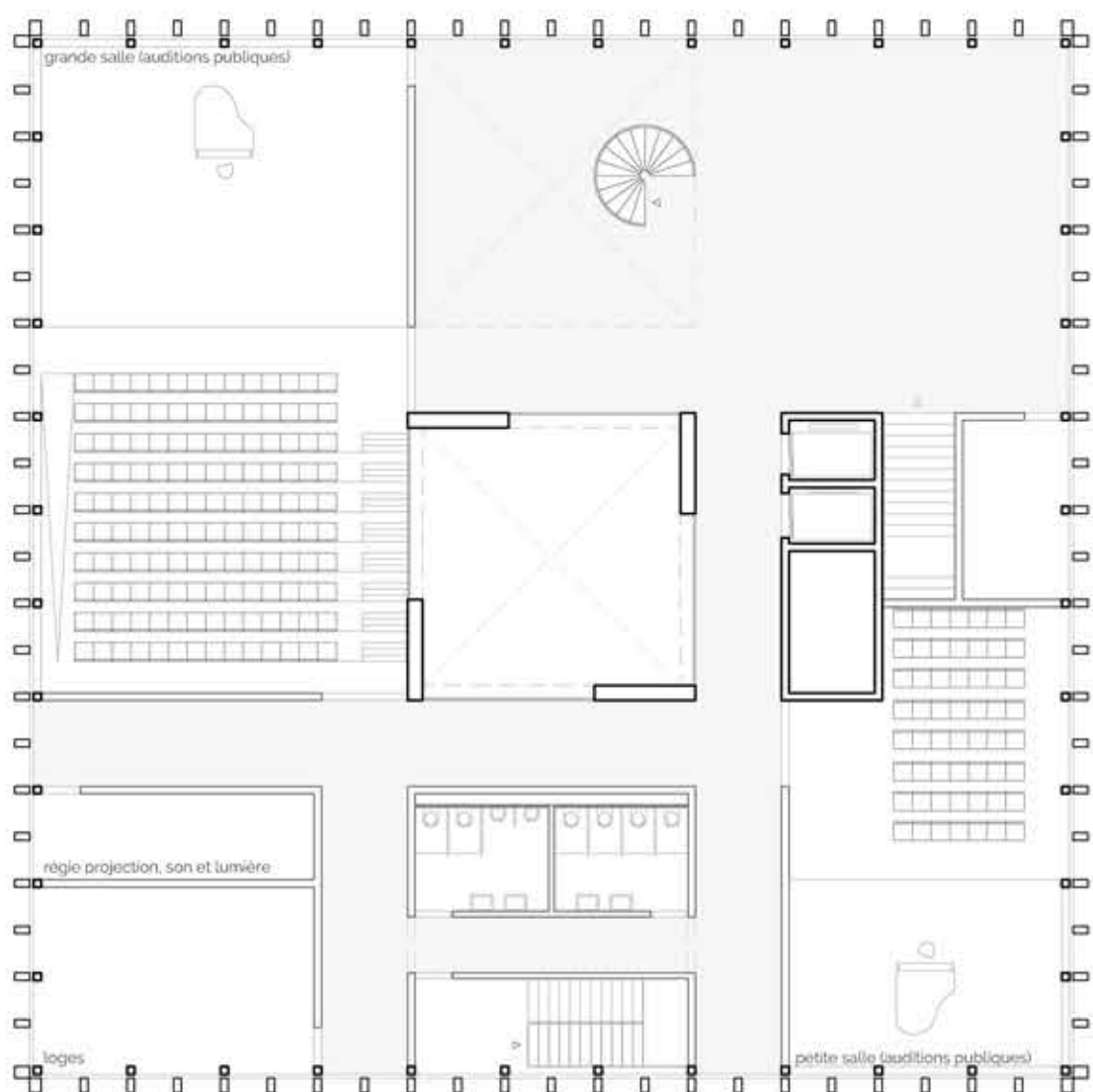
8ème étage salles d'auditions_1:200
