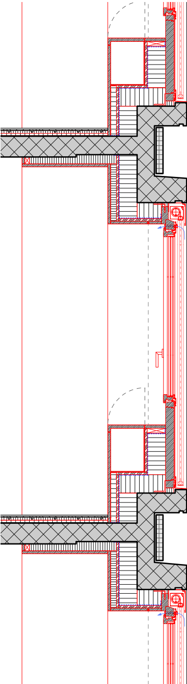
SCHNITT Mst. 1:33
