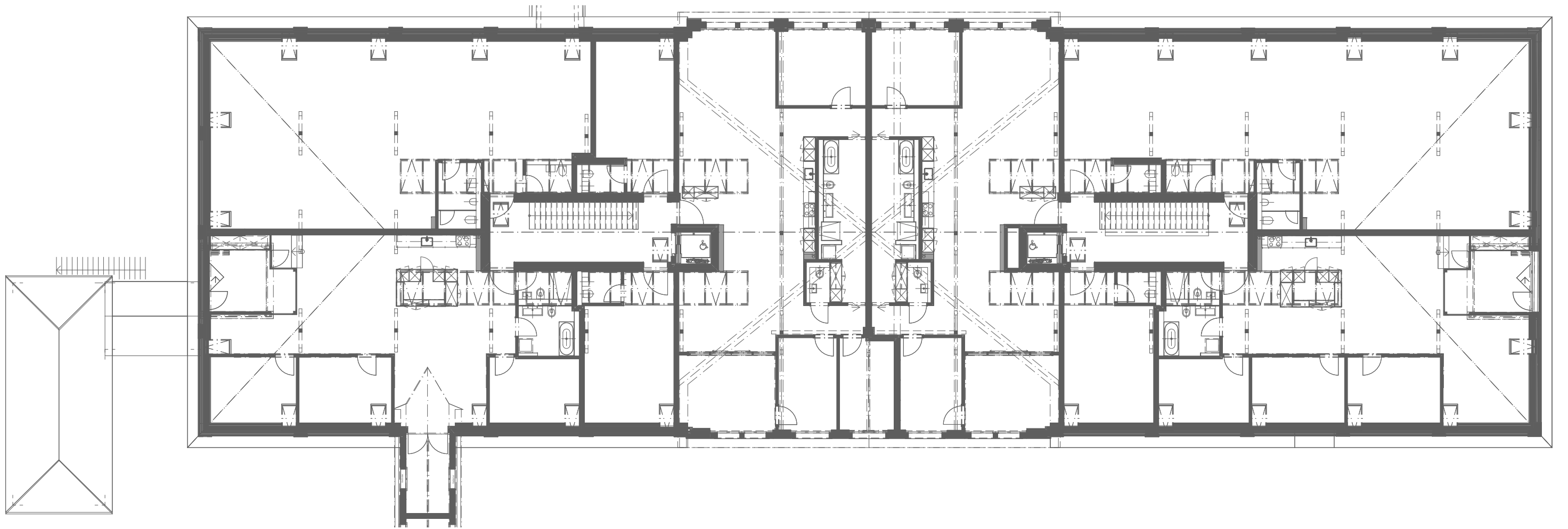
Dachgeschoss
