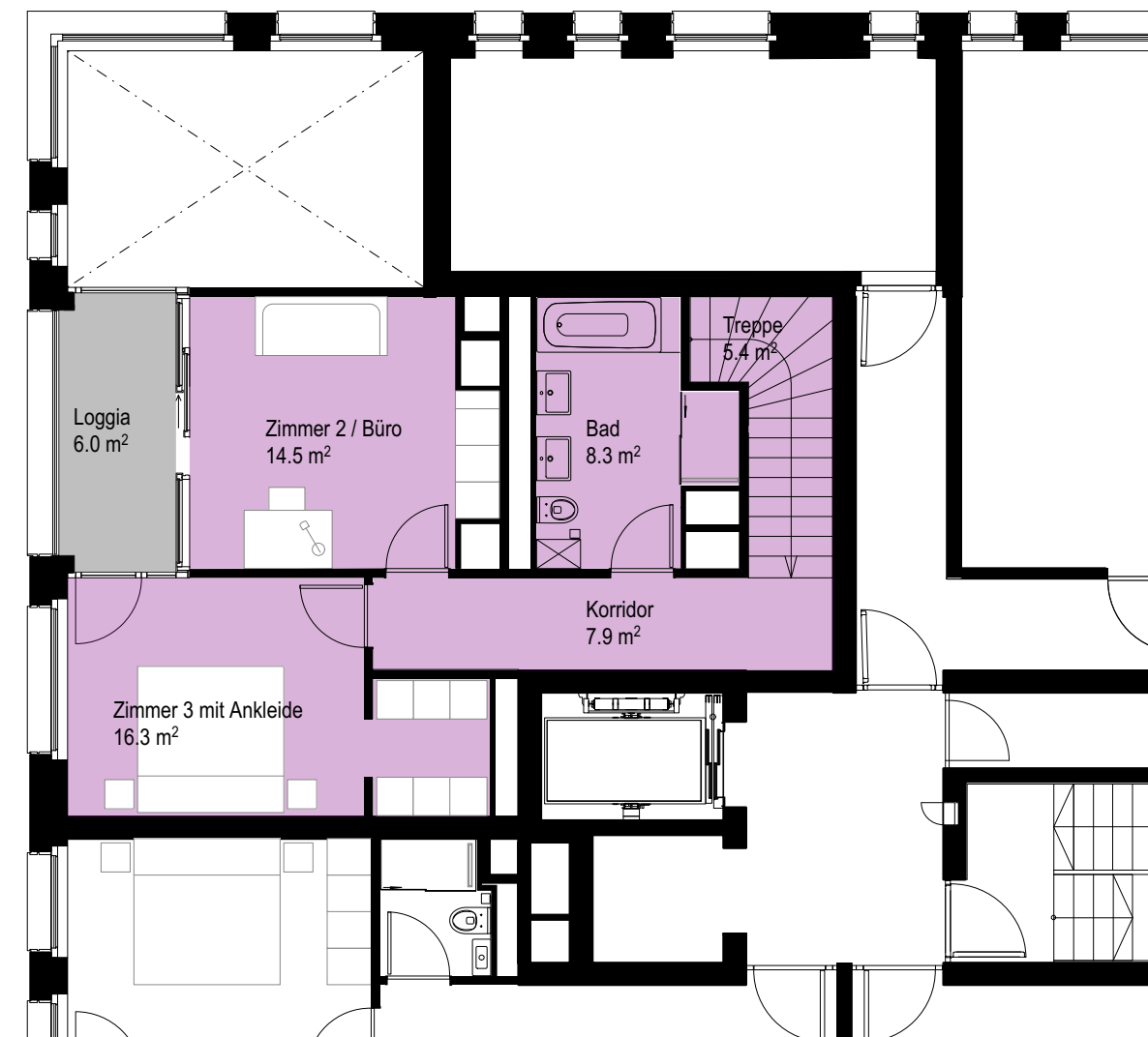
Wohnung A.25.100, MST. 1:100
