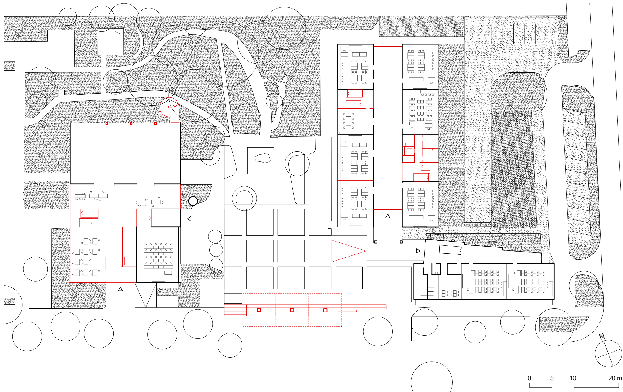
Grundriss Erdgeschoss
