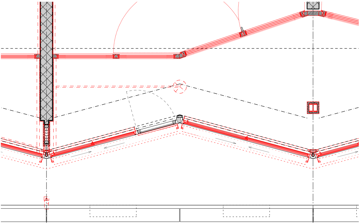
GRUNDRISS Mst. 1:33
