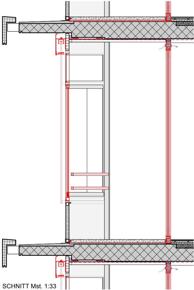
SCHNITT Mst. 1:33
