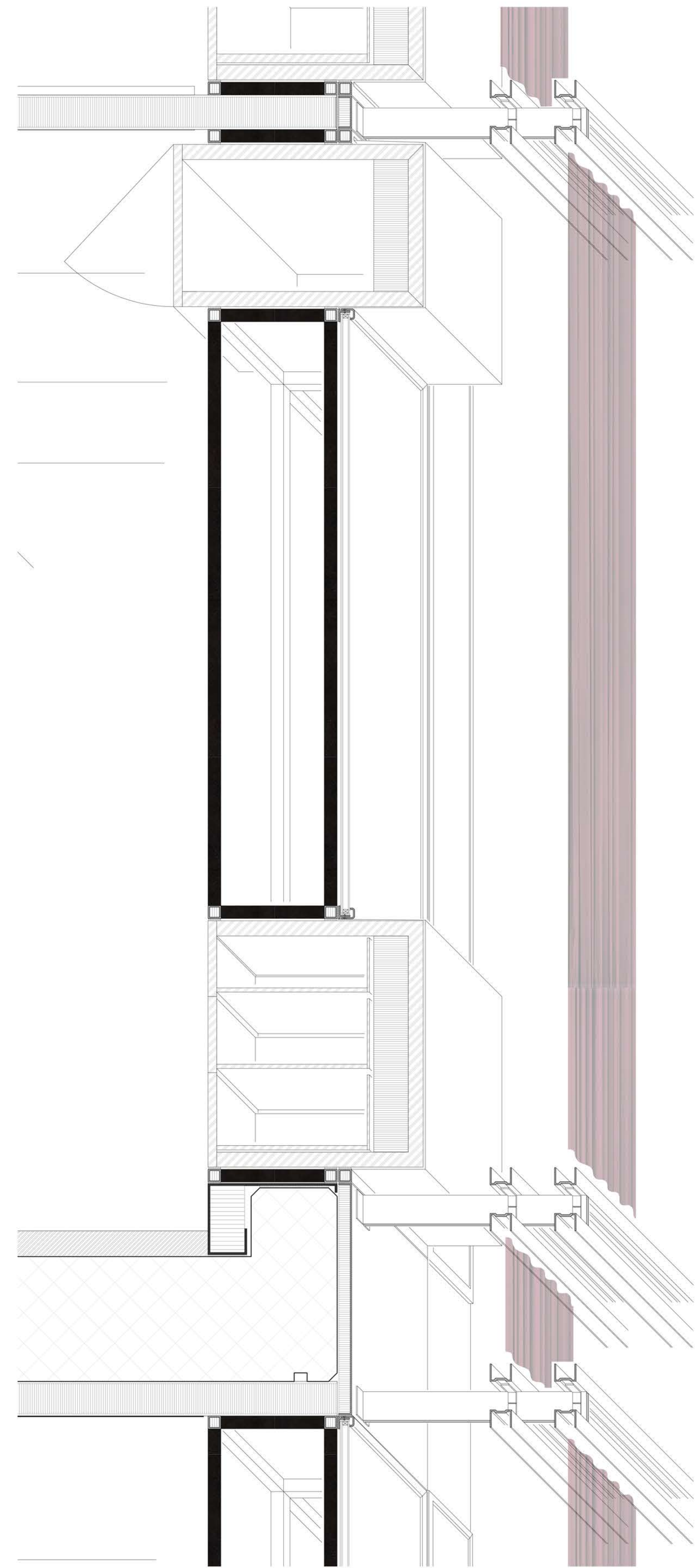
_Fassadenschnitt 1:5
