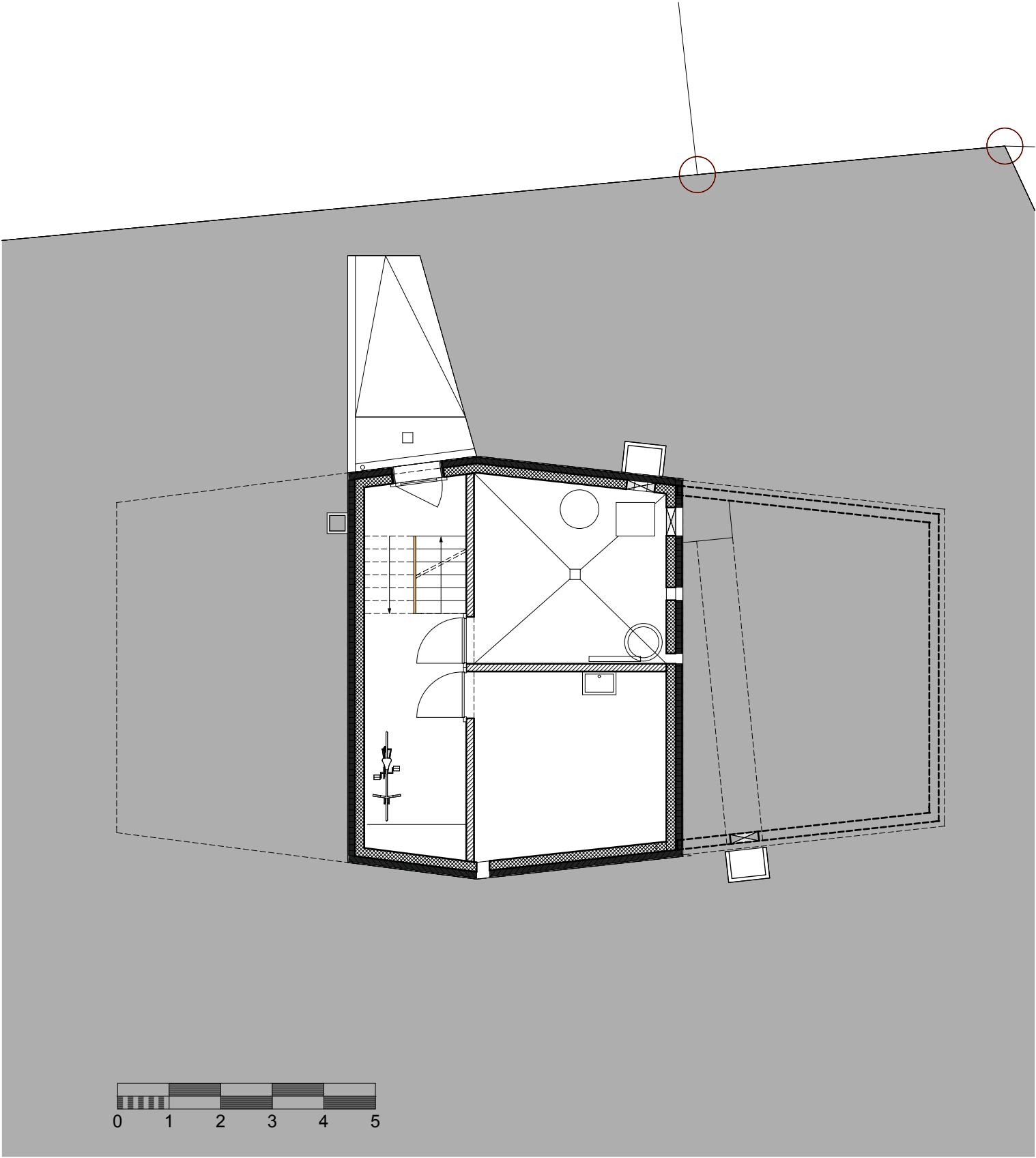
SOUS - SOL
