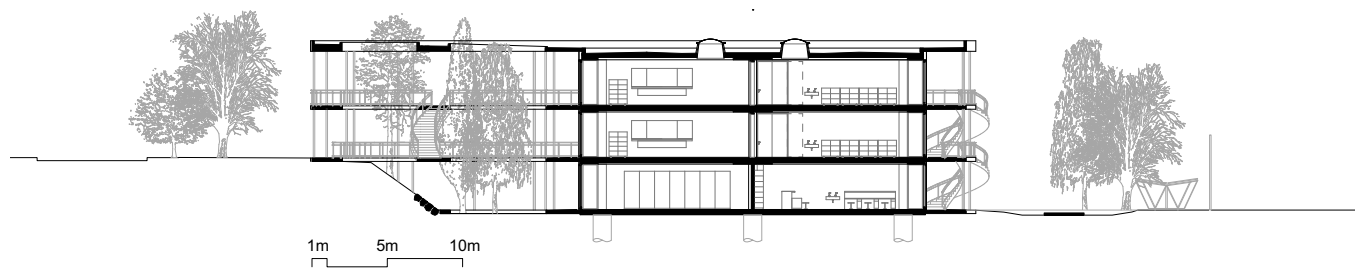
Längsschnitt A-A 1: 500
