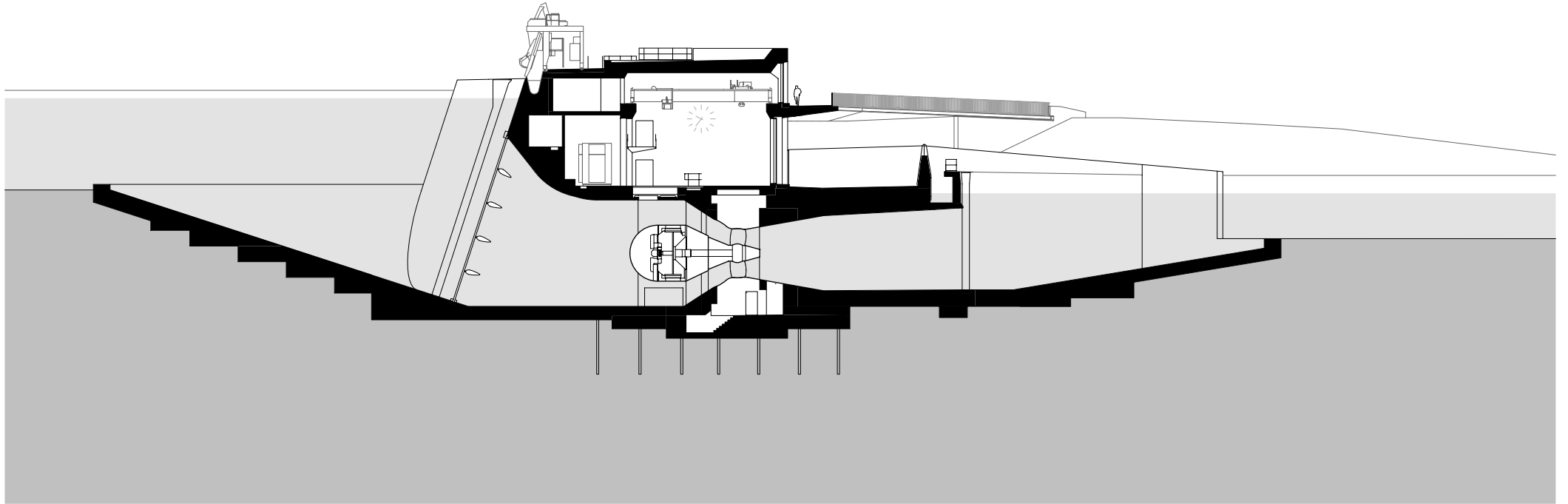
1:500 Schnitt_Turbine
