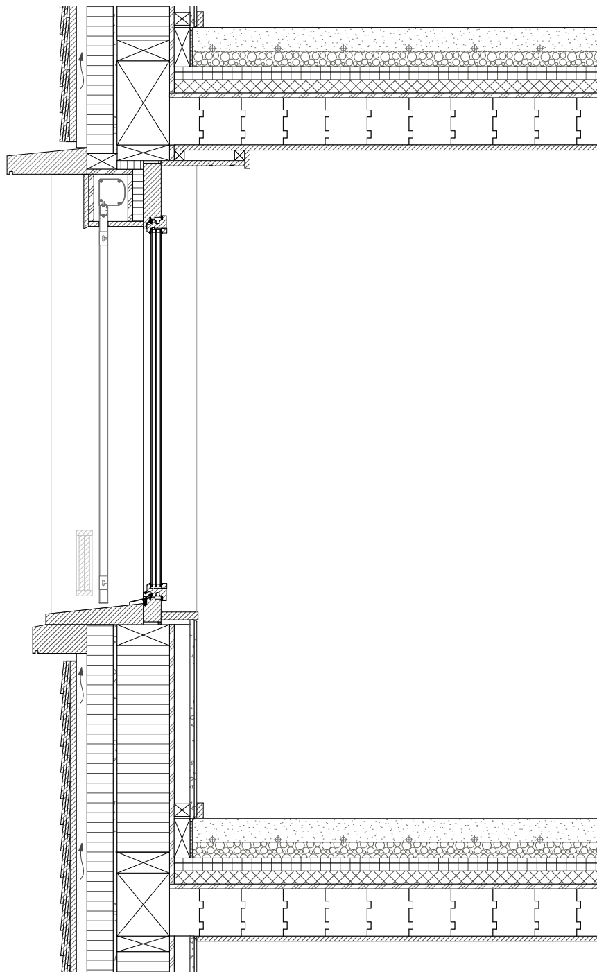
Schnitt
