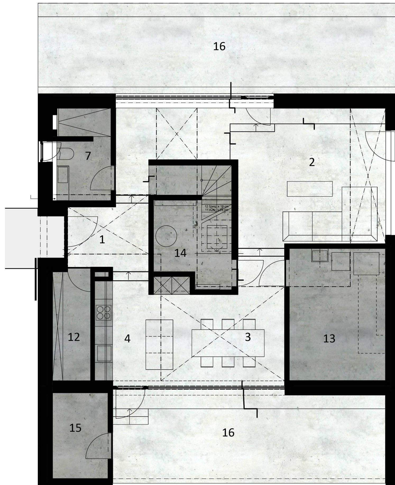
Erdgeschoss
