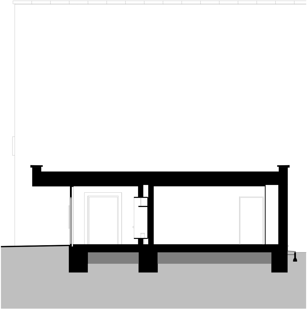
SCHNITT B - 1:100
