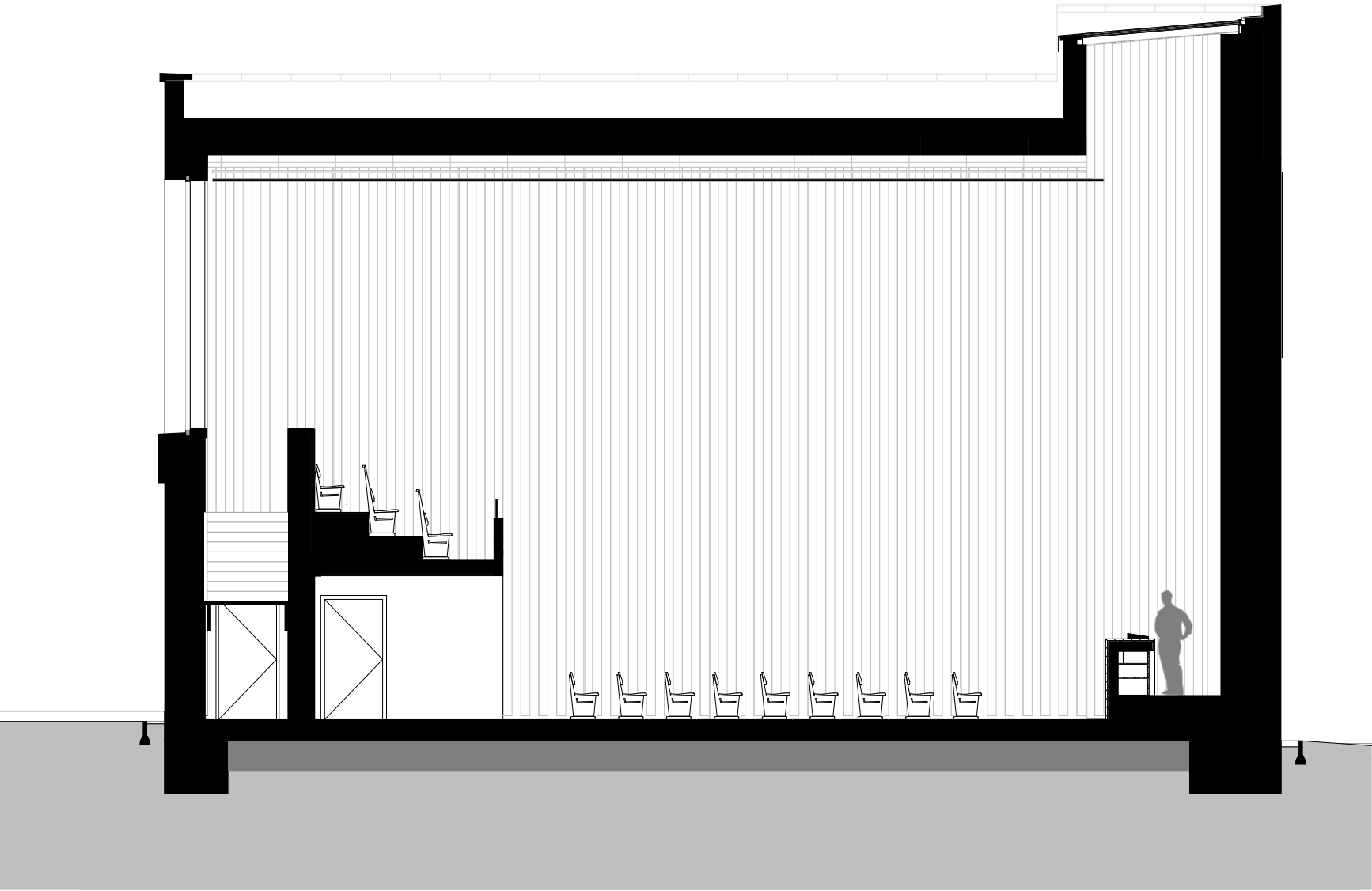
SCHNITT A - 1:100
