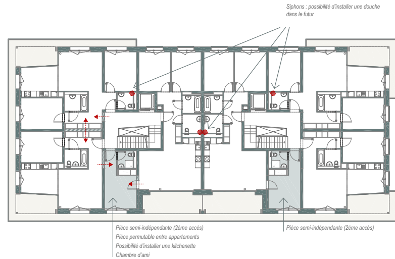
Pièces multifonctionnelles et flexibilité de l'étage type
