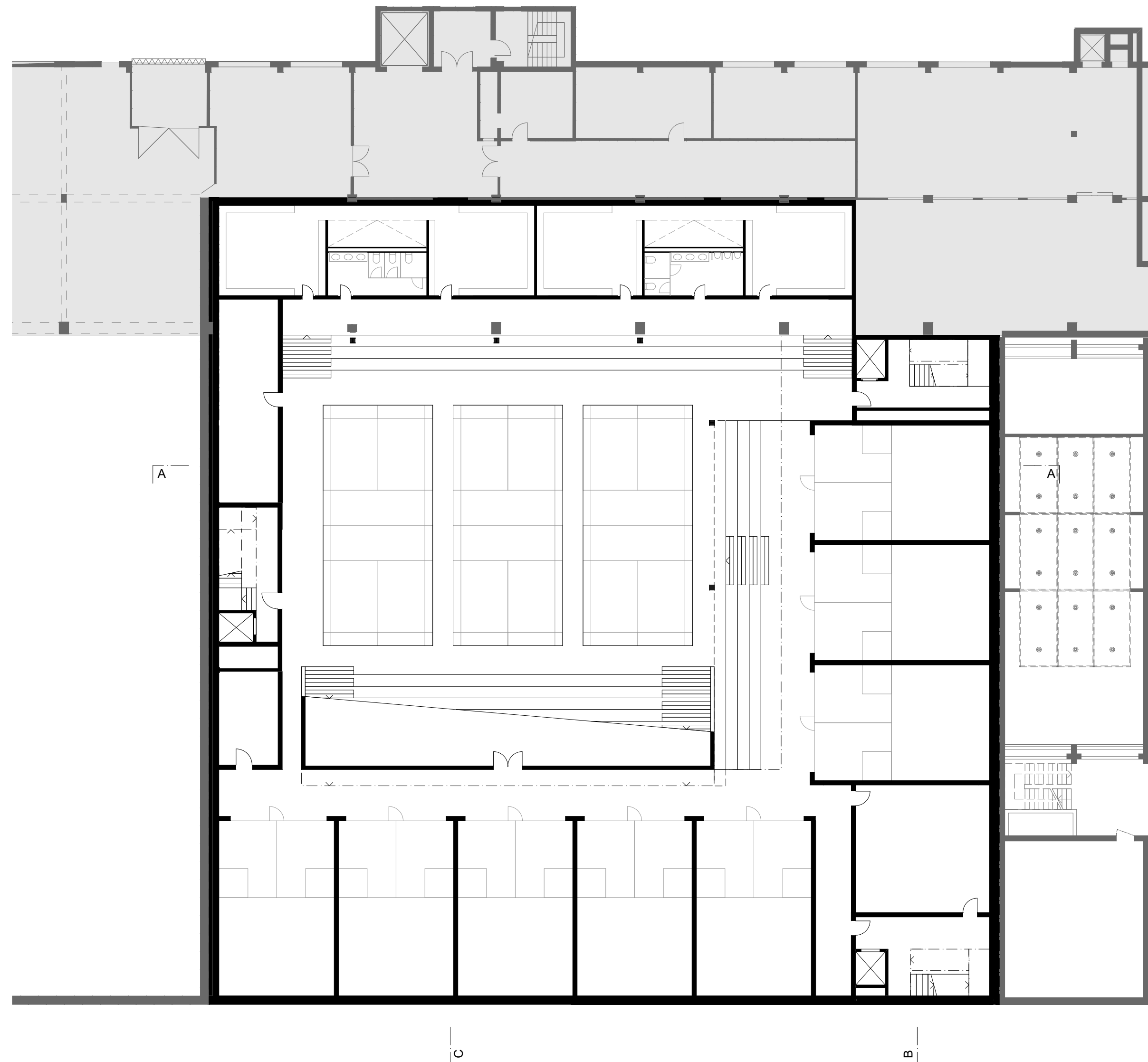
Grundriss Untergeschoss 1:200
