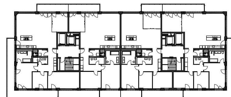
1./3./5./7./9. Obergeschoss
