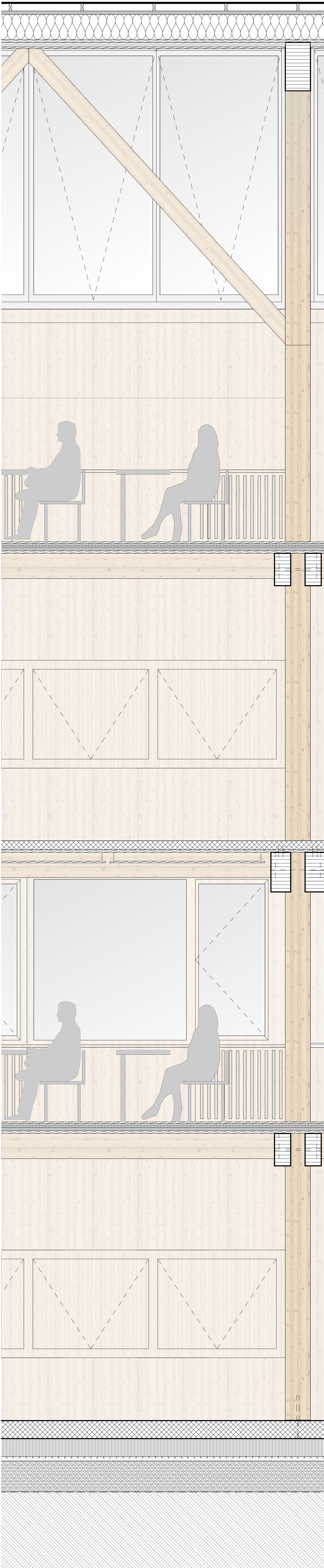
Vue intérieure - 1:20
