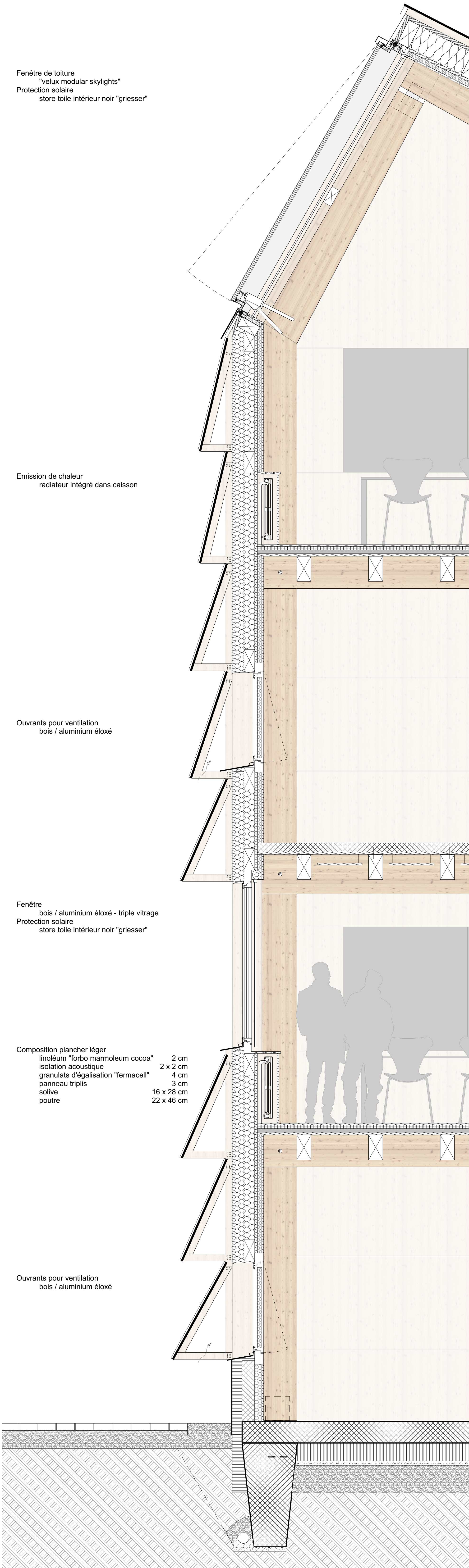
Travée Nord - 1:20
