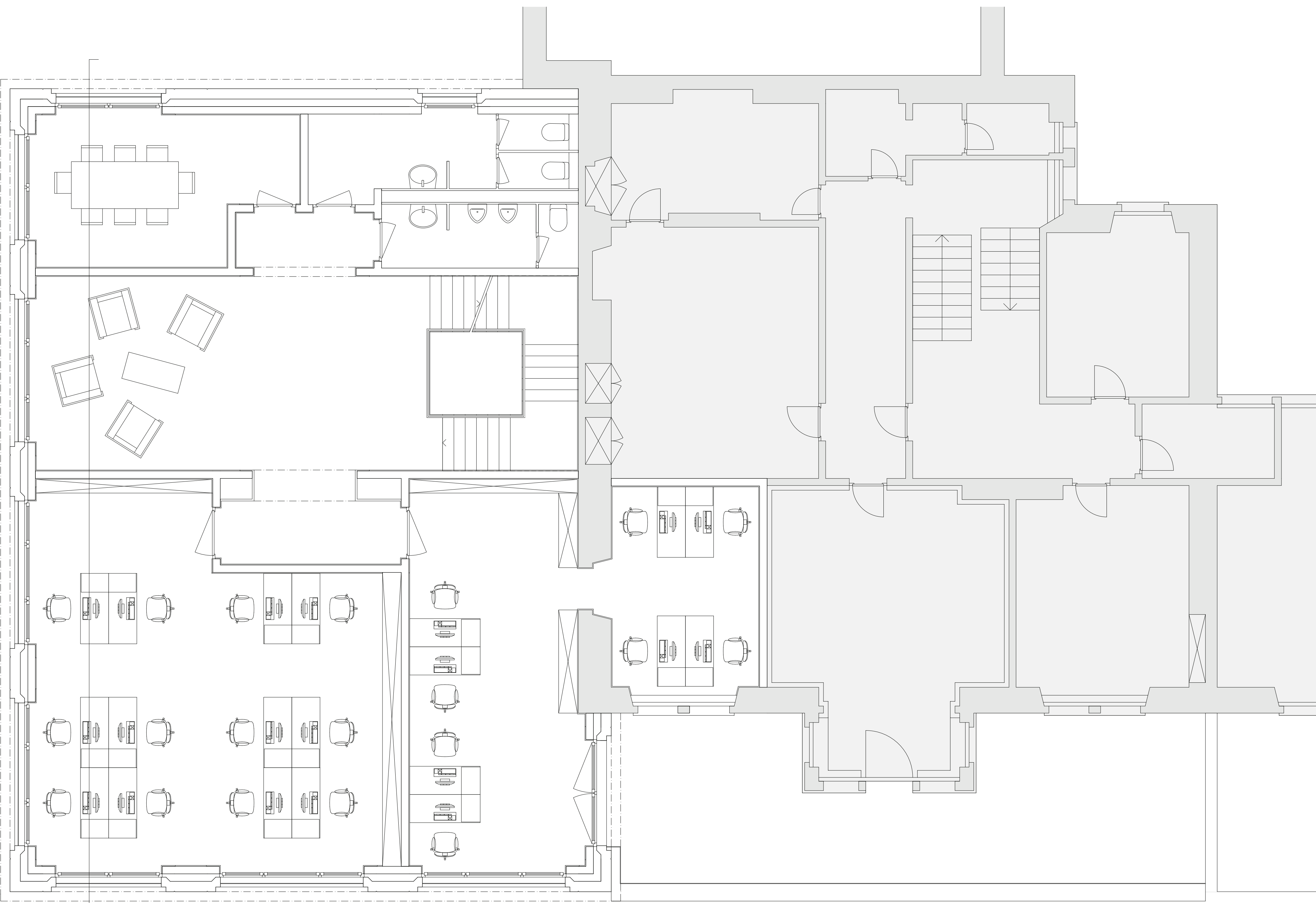
Grundriss Obergeschoss 1:50
