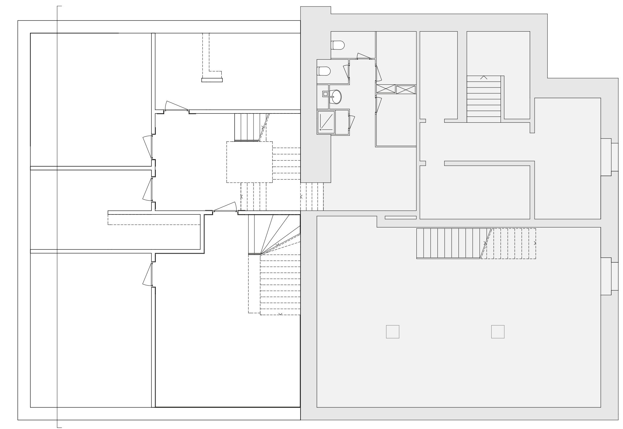
Grundriss Untergeschoss 1:100
