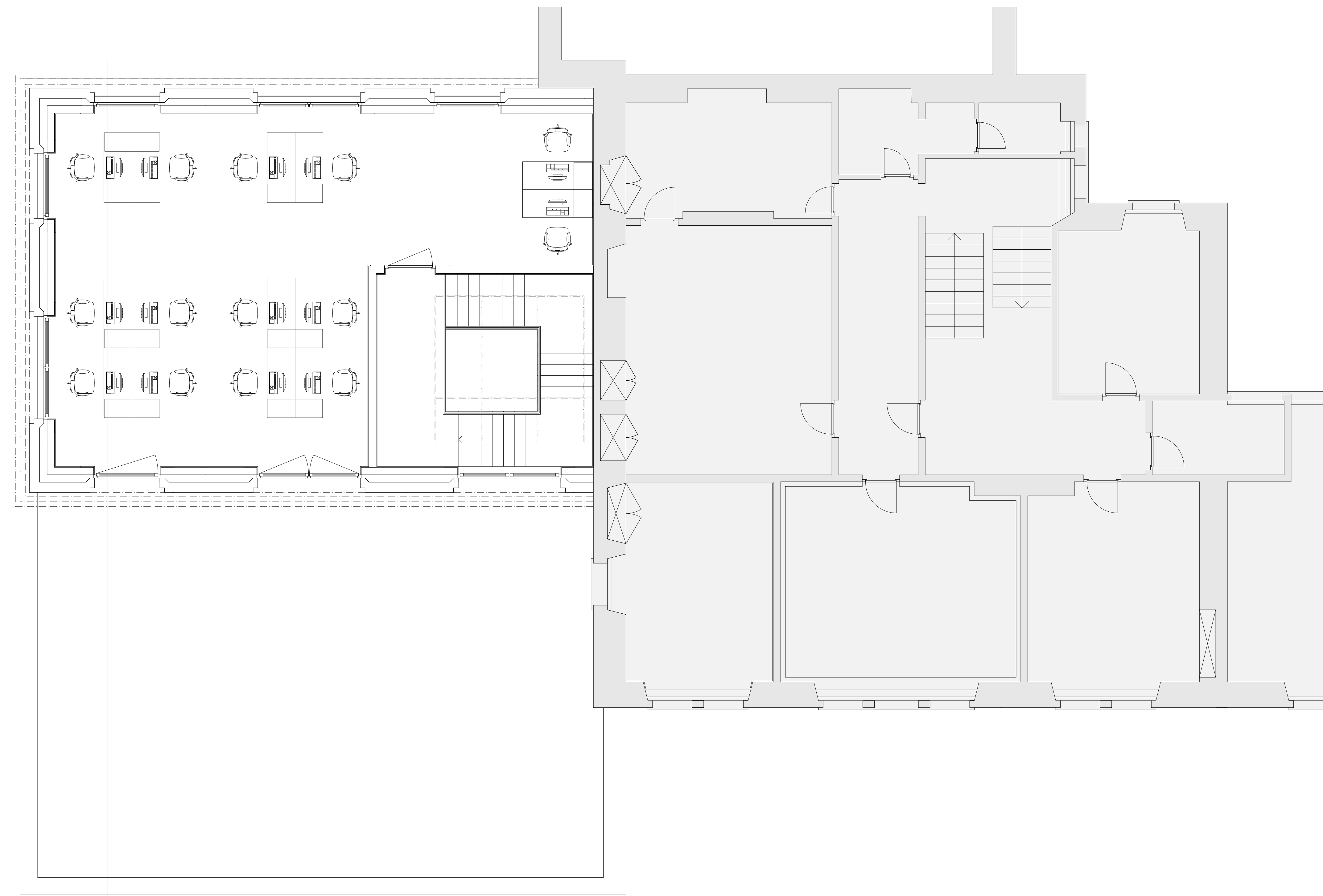
Grundriss Dachgeschoss 1:50
