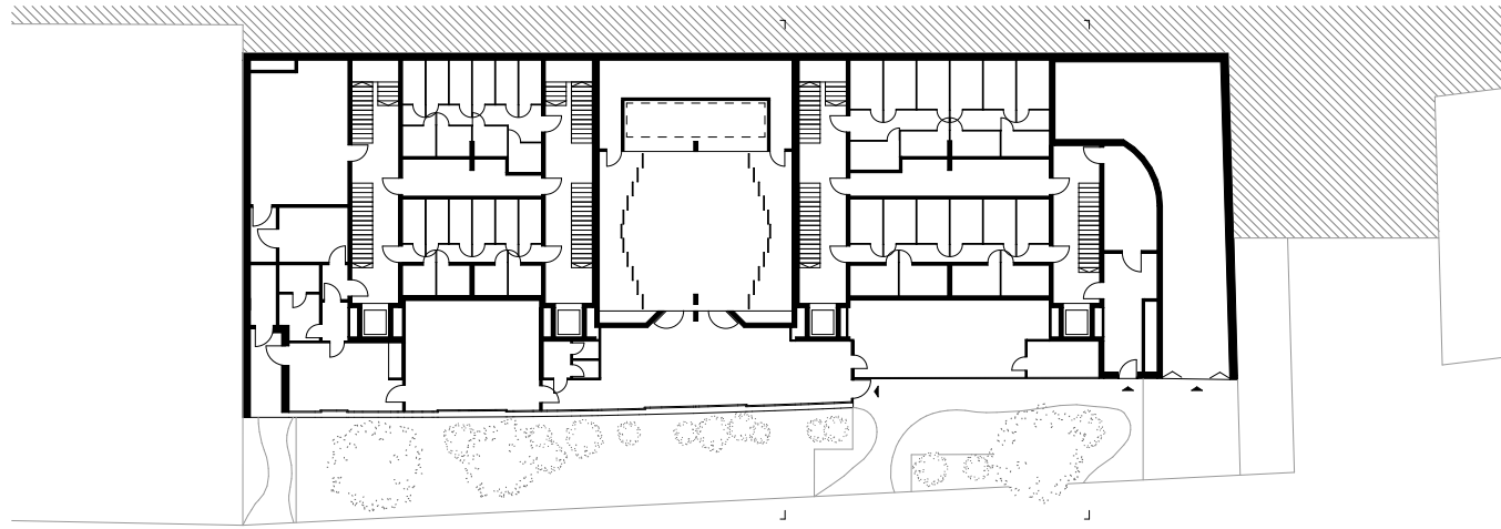
Rez-de-chaussée
