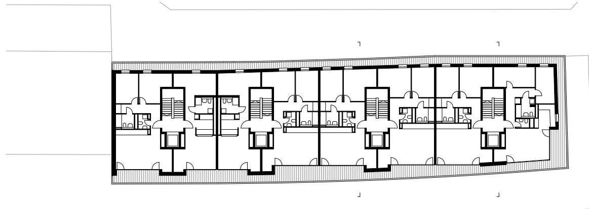
Attique
