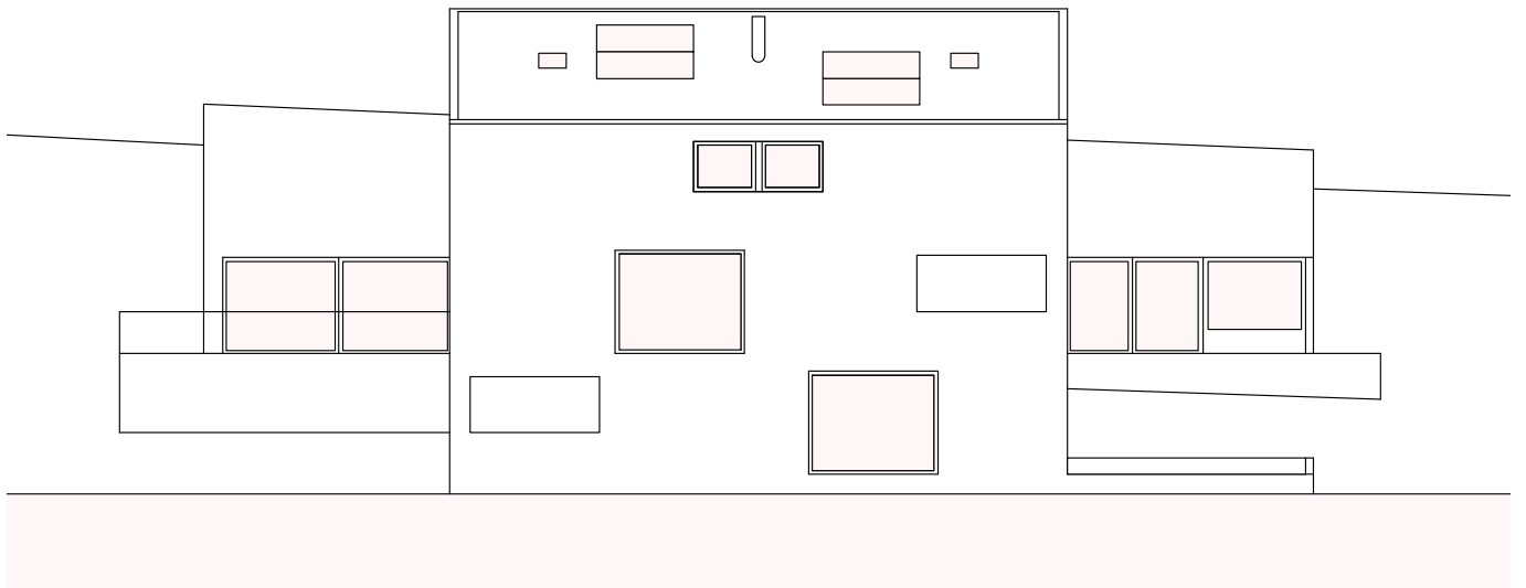
COUPE E-E
