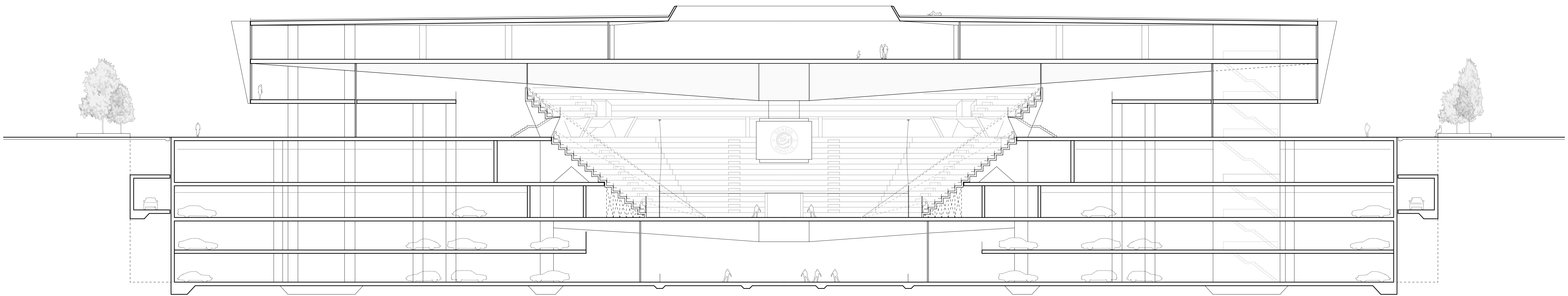
coupe transversale ech. 1/250
