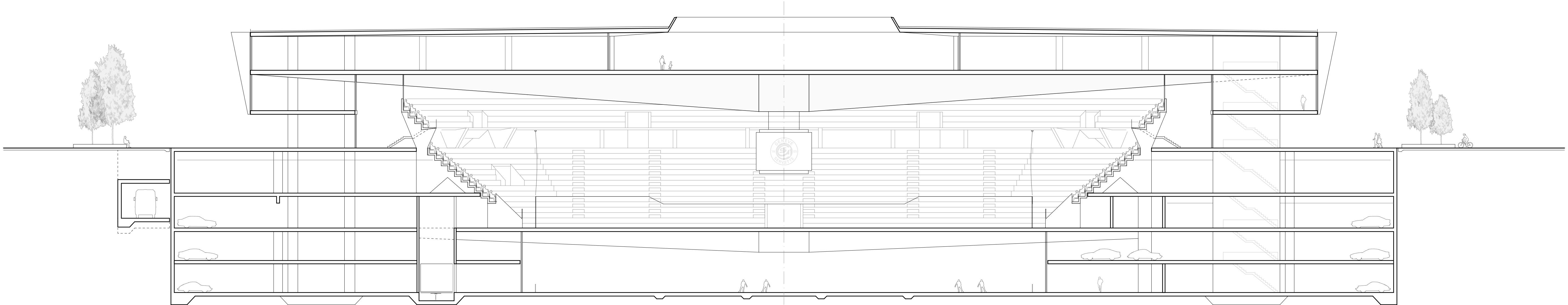
coupe longitudinale ech. 1/250
