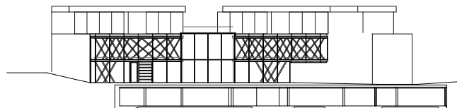
Elévation Est
