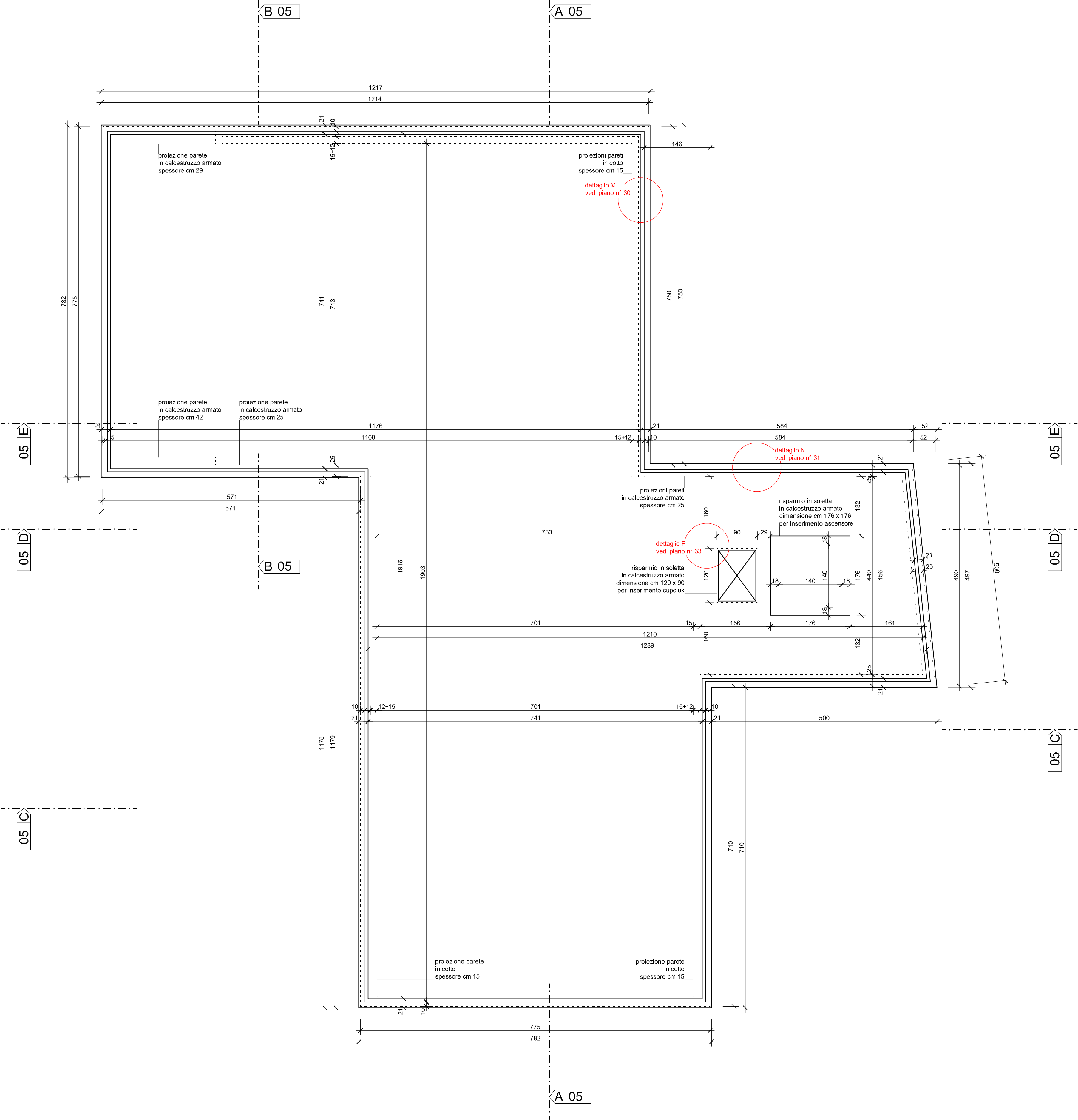
Pianta Piano Tetto 1:50
