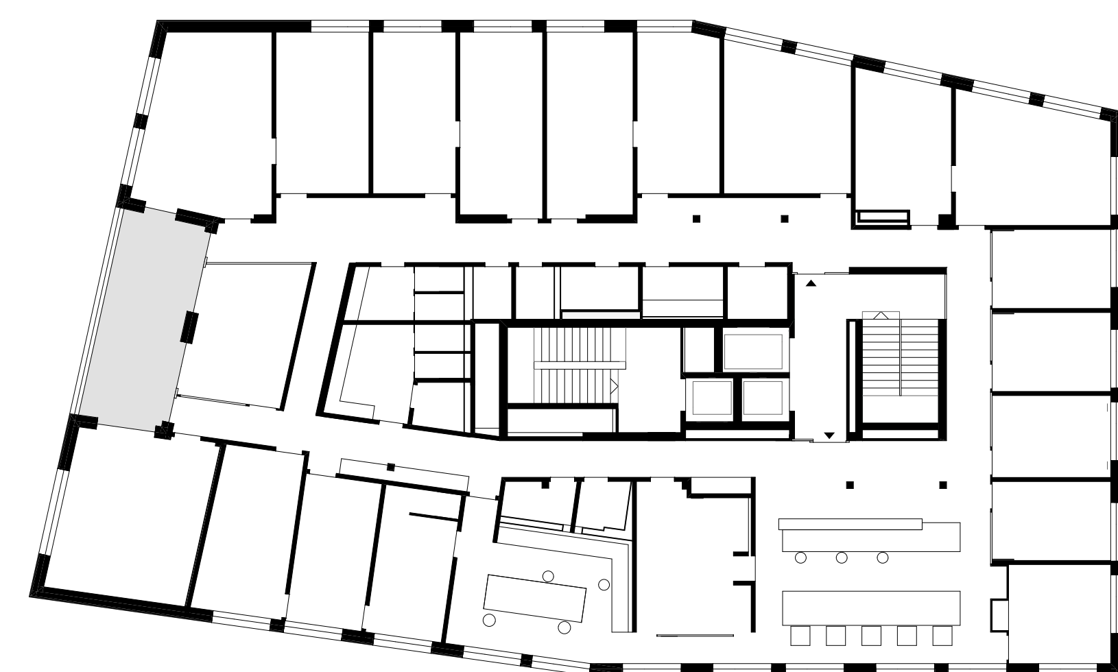
1. Obergeschoss
