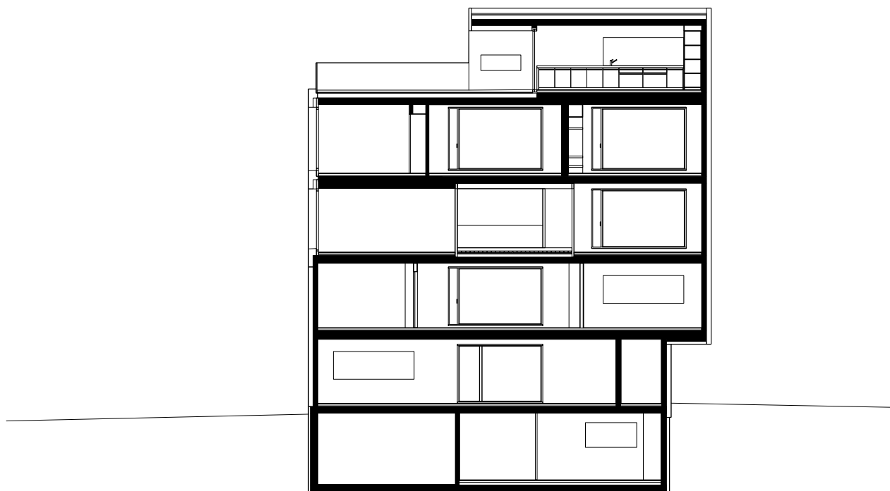
Schnitt 1:200
