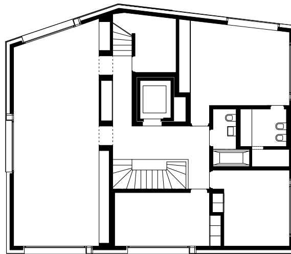
3. Obergeschoss 1:200
