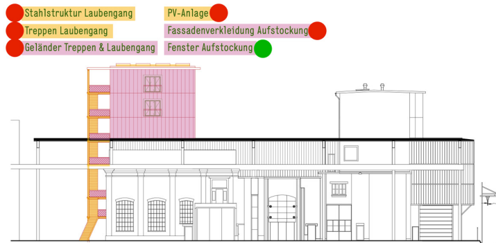
Südwestfassade - zur offenen Halle 142
