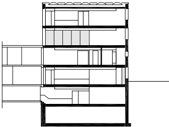
Coupe EE
