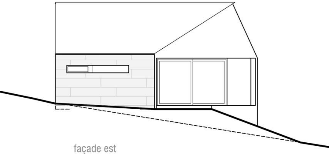
façade est
