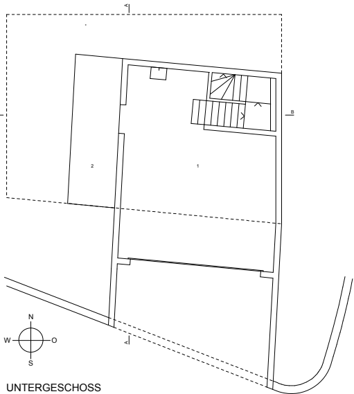
UNTERGESCHOSS
