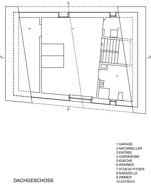
DACHGESCHOSS
