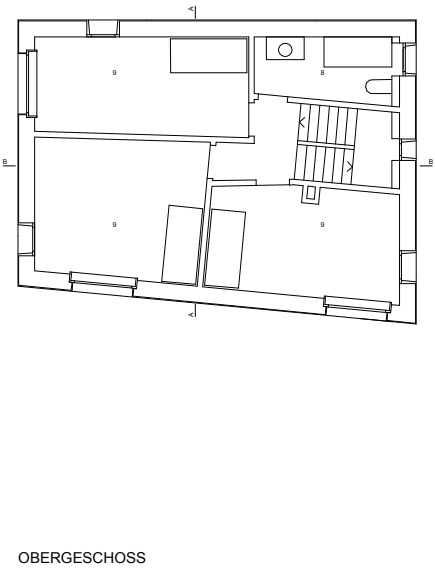
OBERGESCHOSS
