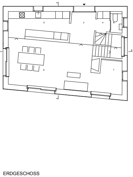
ERDGESCHOSS
