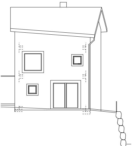
WESTFASSADE
