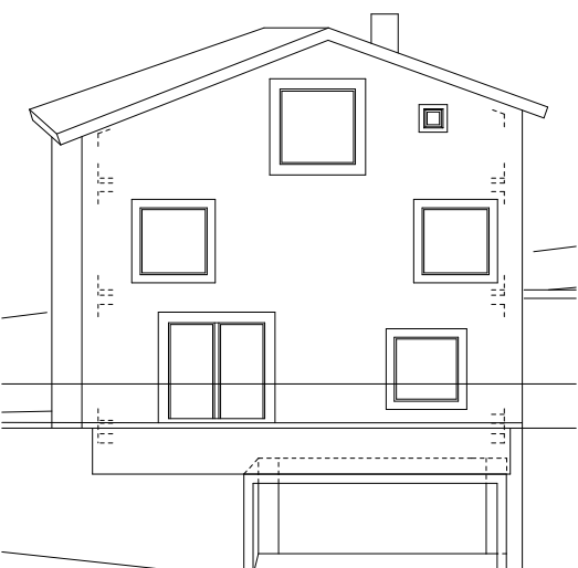
SÜDFASSADE
