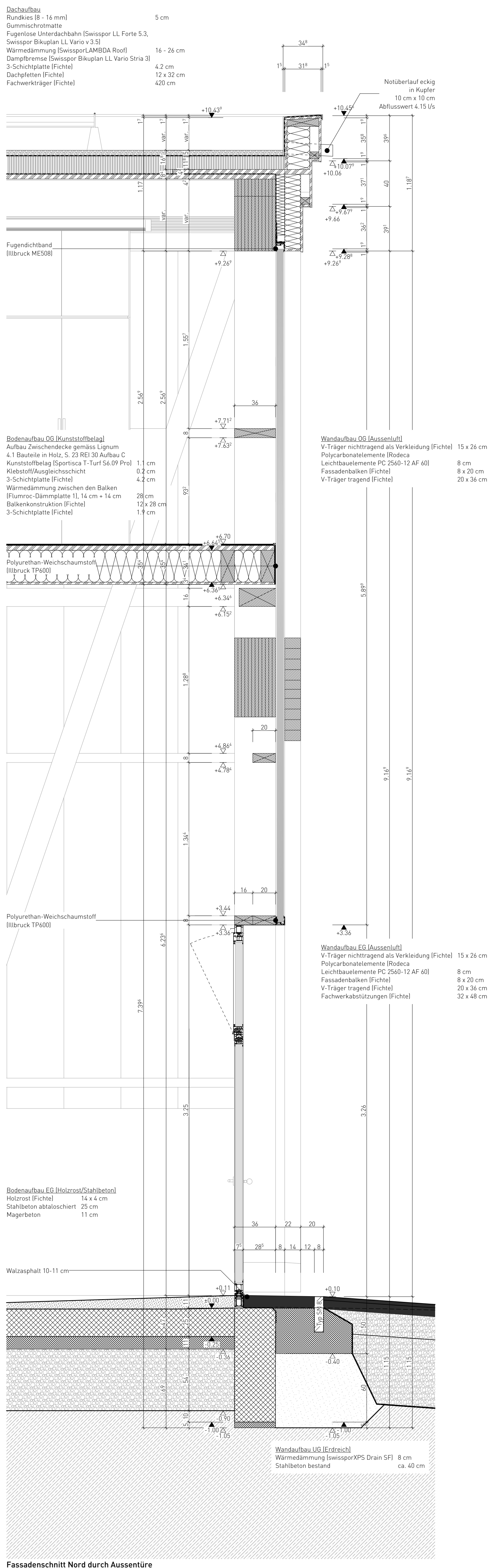
Fassadenschnitt Nord durch Aussentüre
