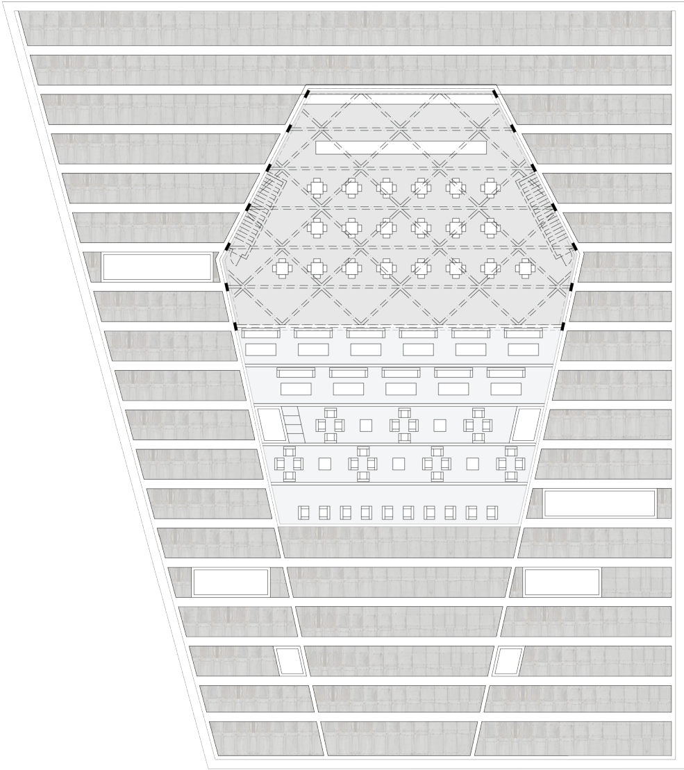
Dachaufsicht 1:200
