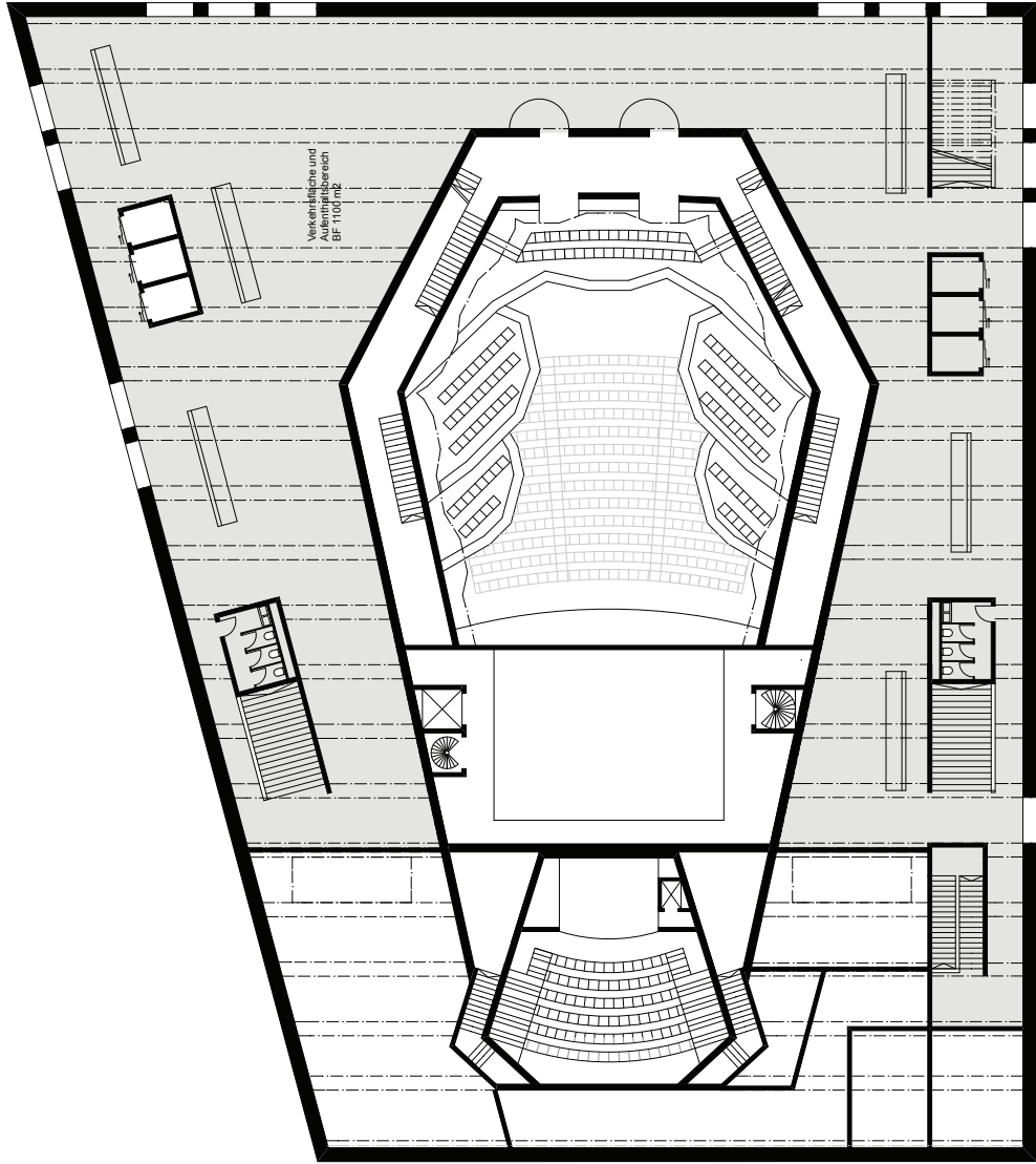
3. Obergeschoss 1:400
