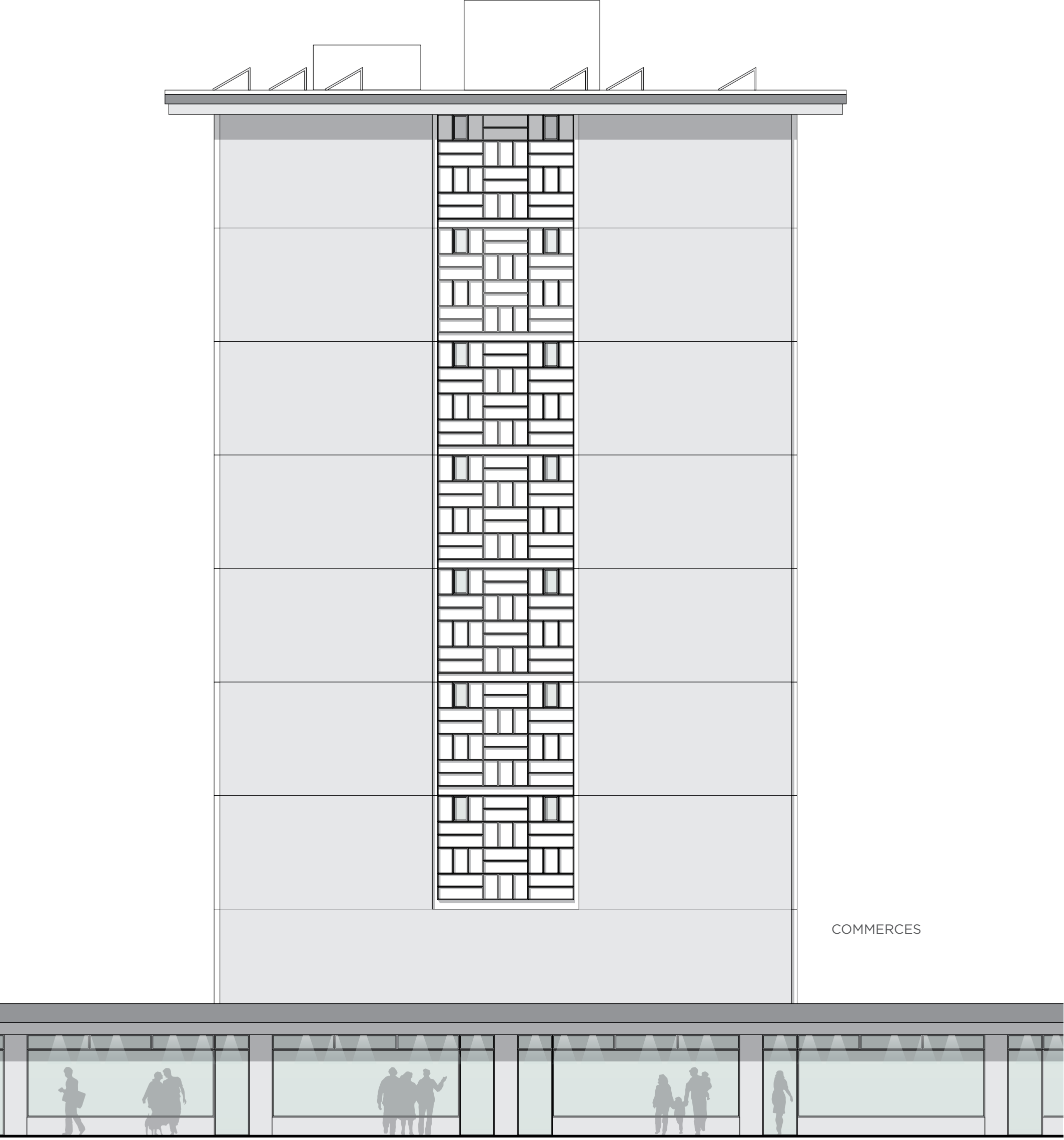
FAÇADE BOULEVARD CARL-VOGT
