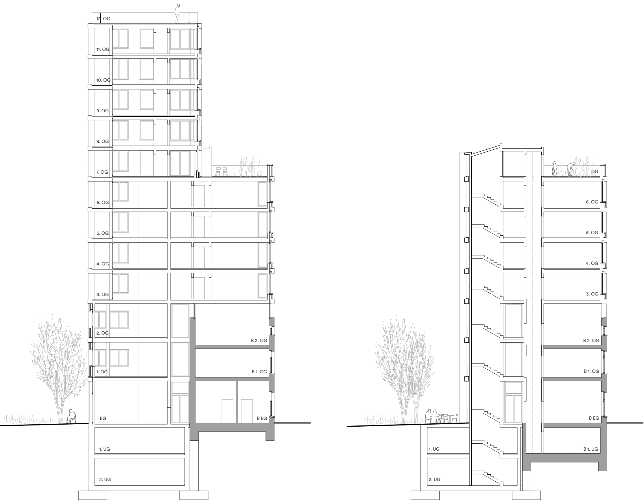
querschnitte wohnhaus
