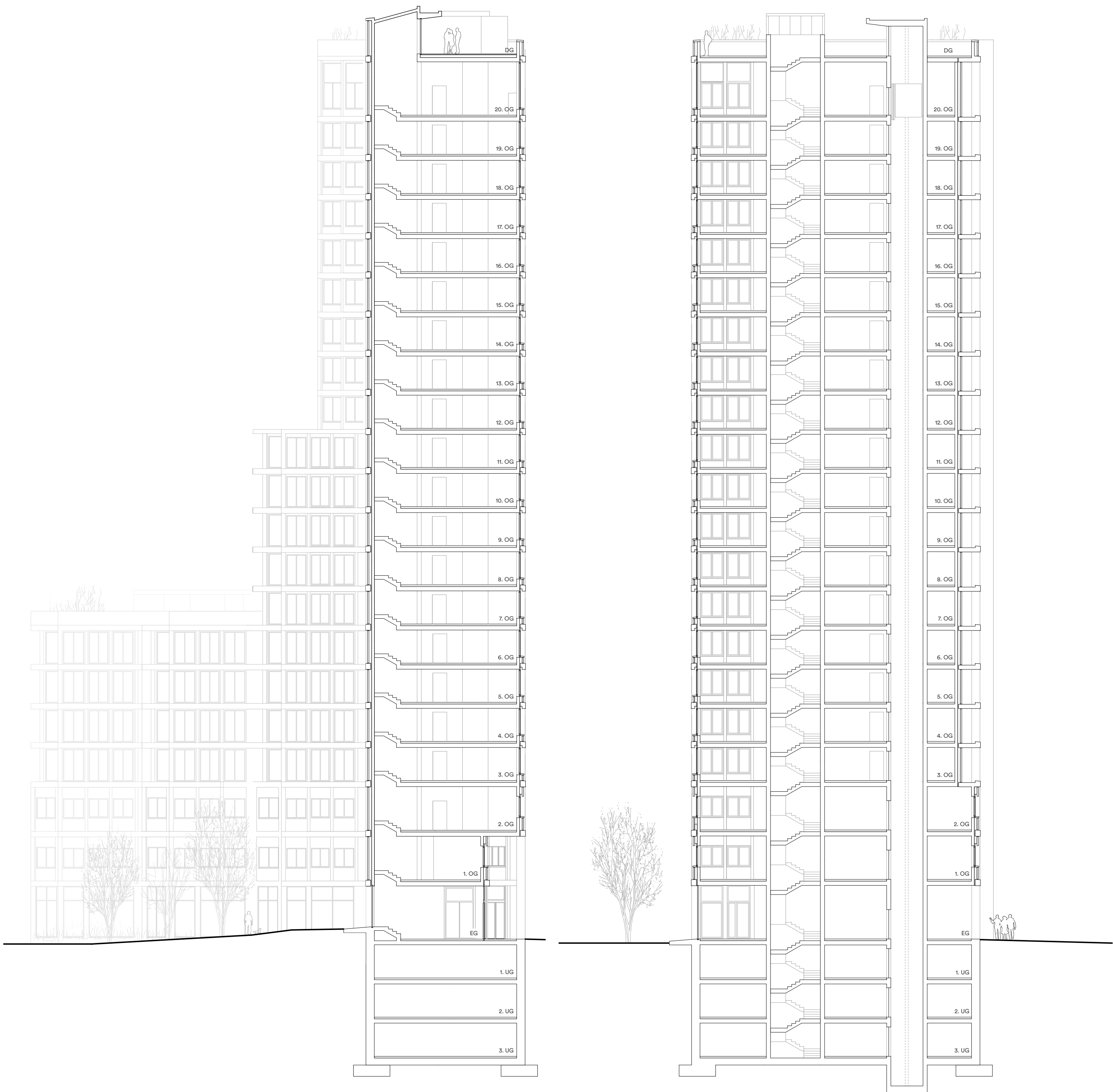
ansicht S-O
