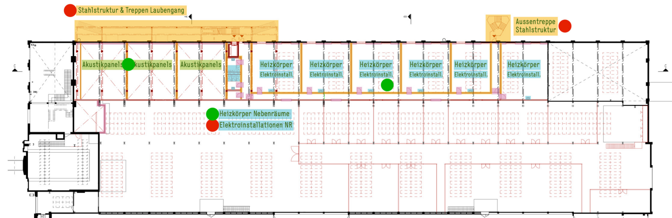
Grundriss 2.OG
