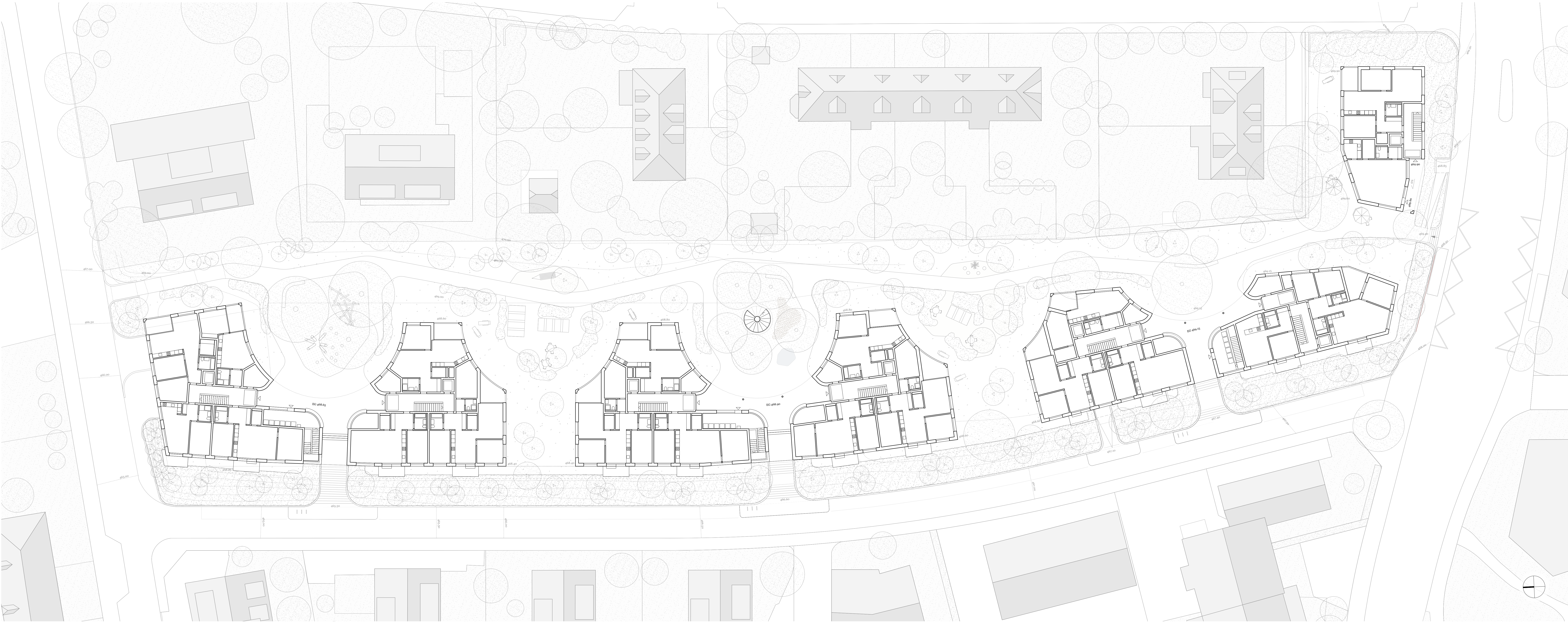
Grundriss Erdgeschoss 1:200
