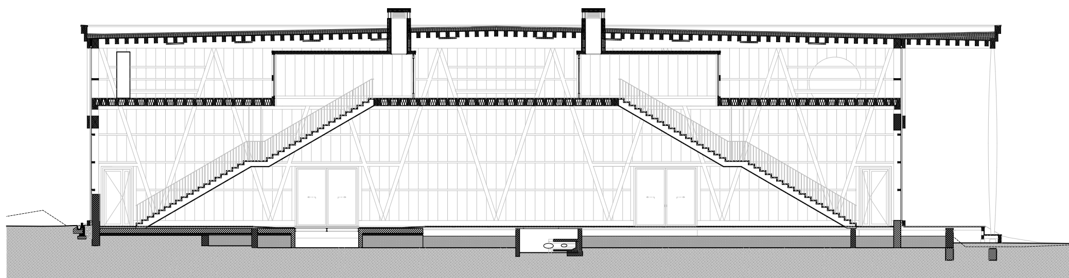
Schnitt E-E
