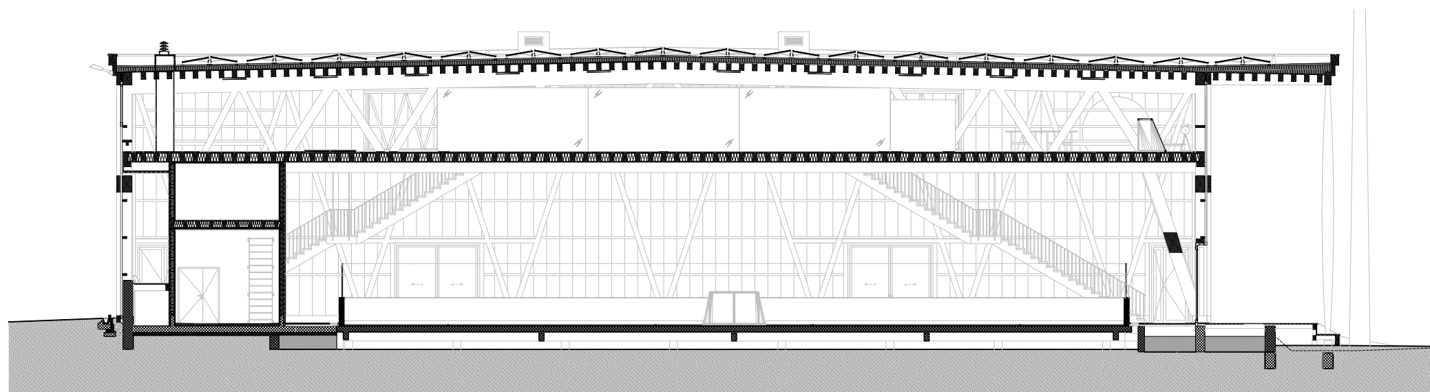
Schnitt D-D
