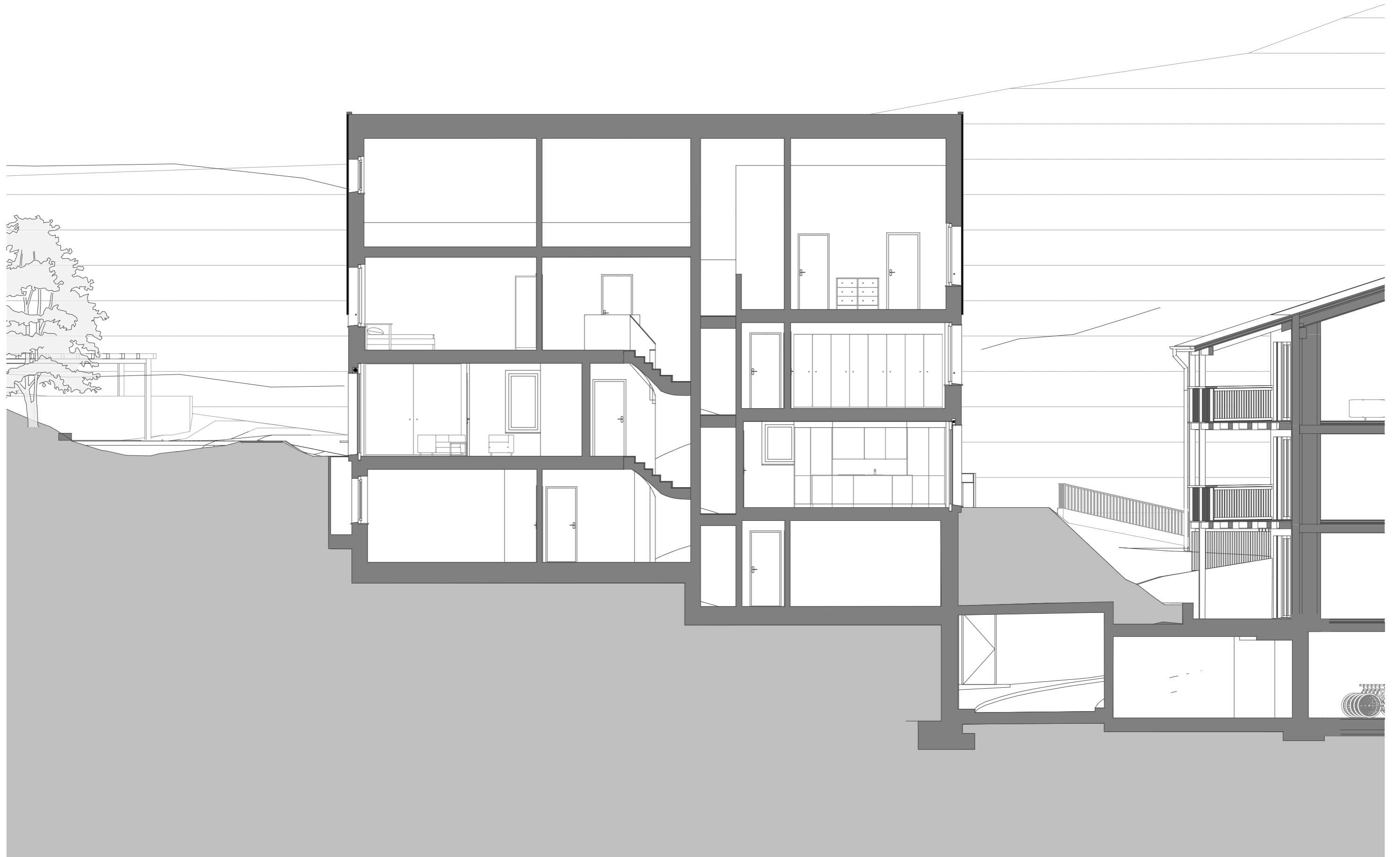
SCHNITT III DEFH / 1:100
