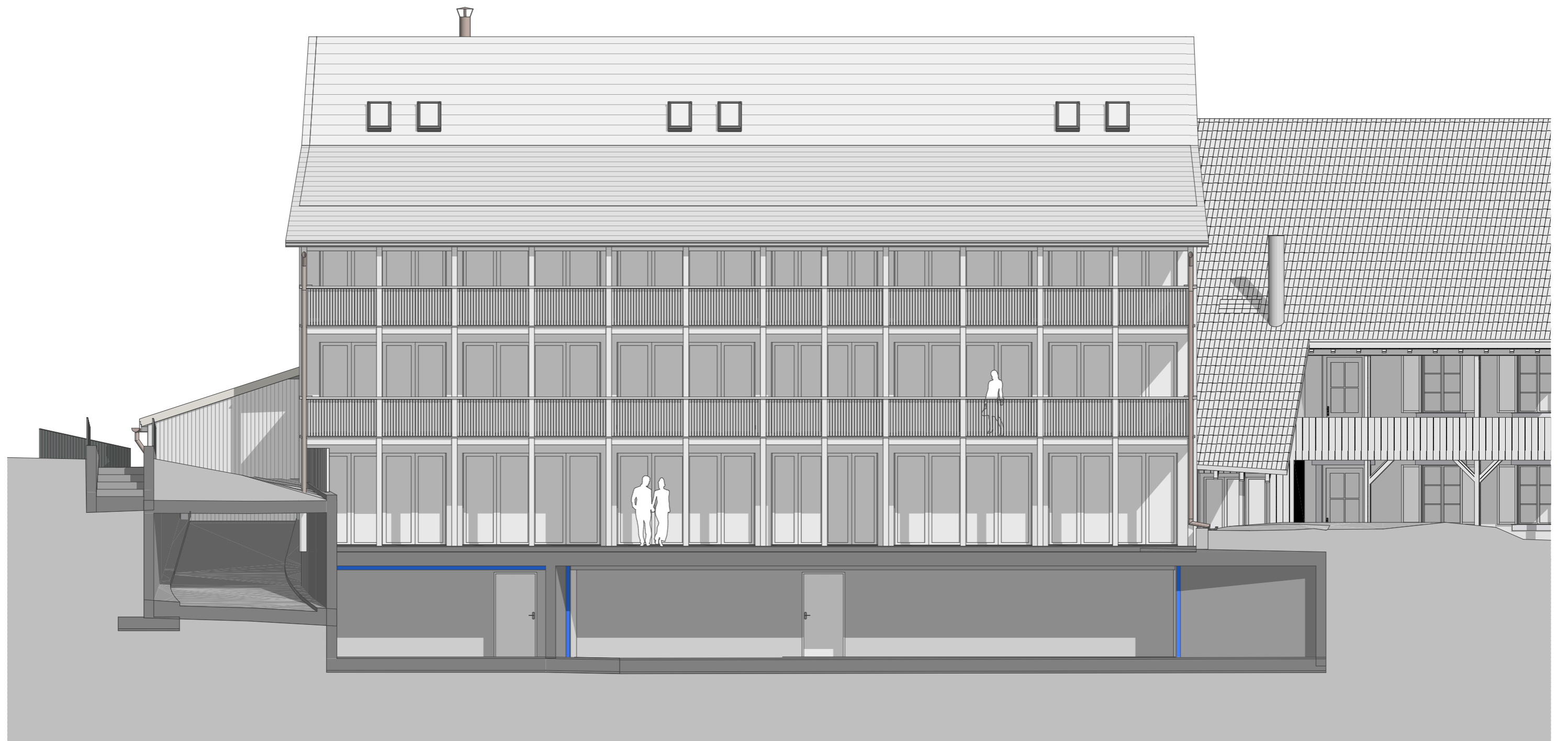
ANSICHT MFH WEST / 1:100
