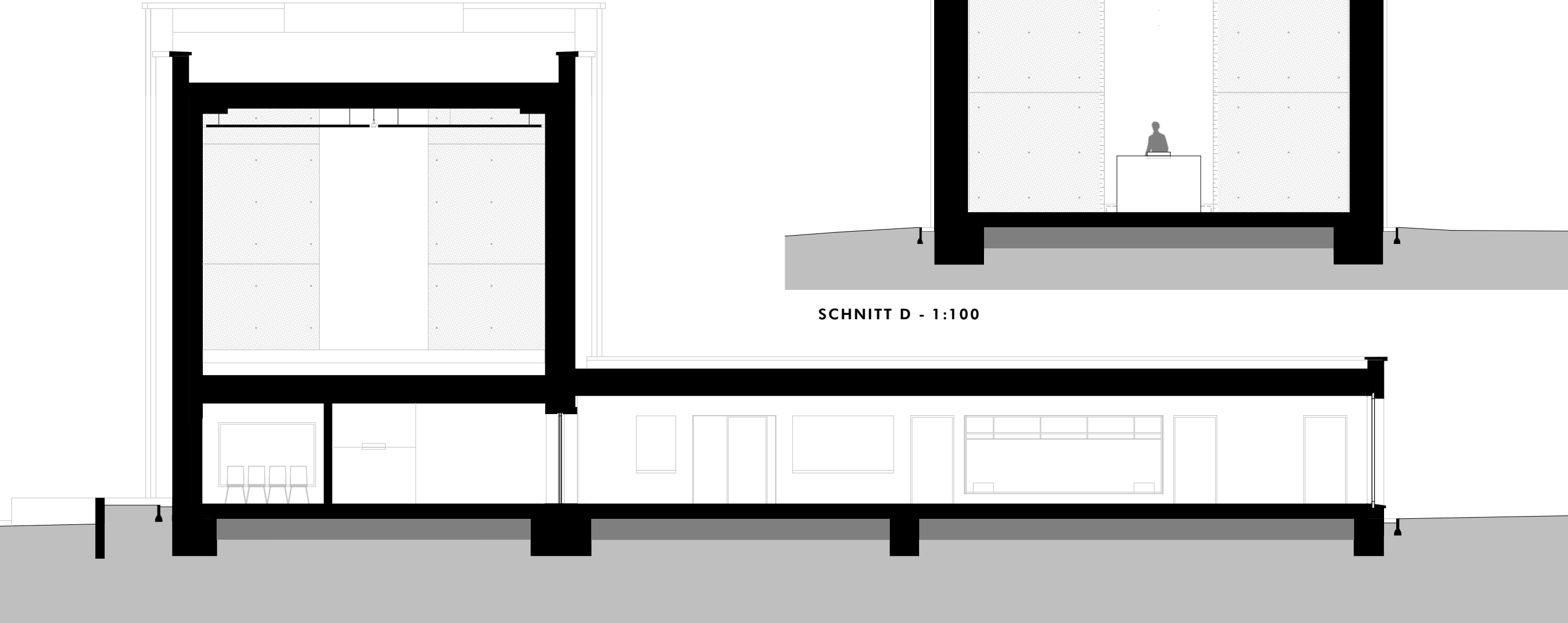
SCHNITT C - 1:100
