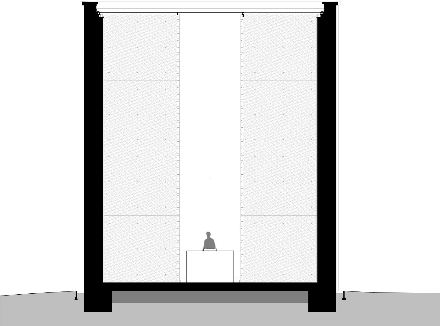
SCHNITT D - 1:100
