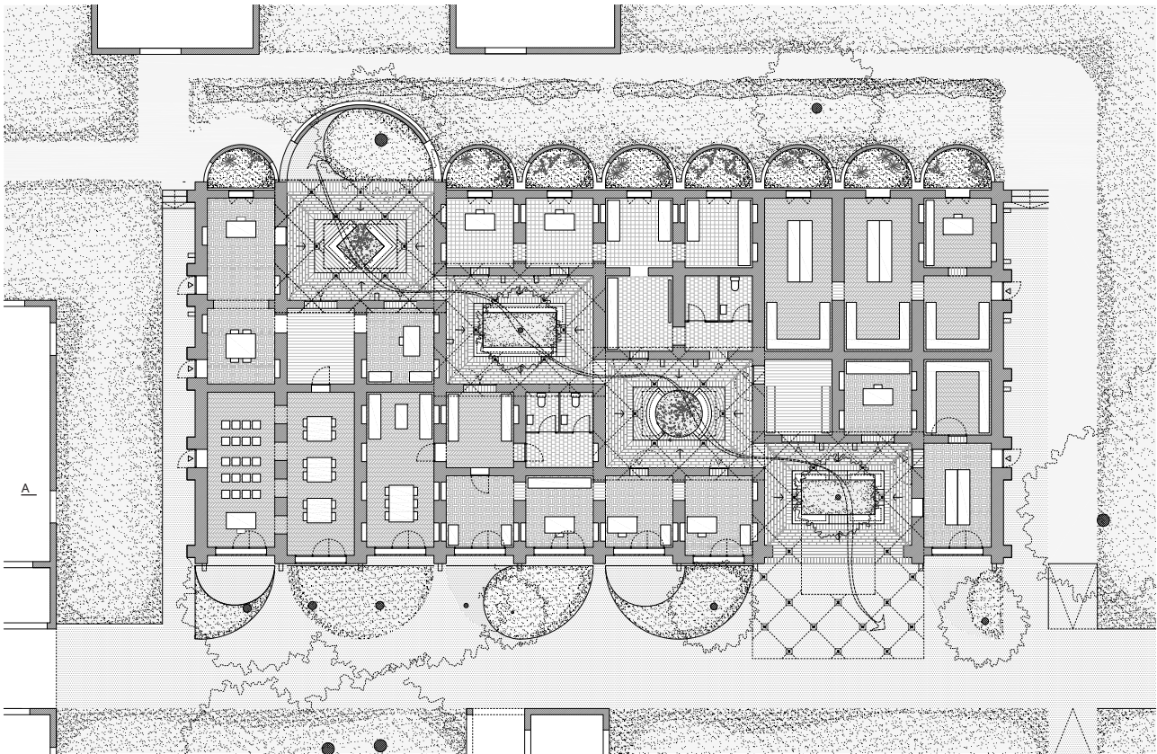
Erdgeschoss | Rez-de-chaussée
