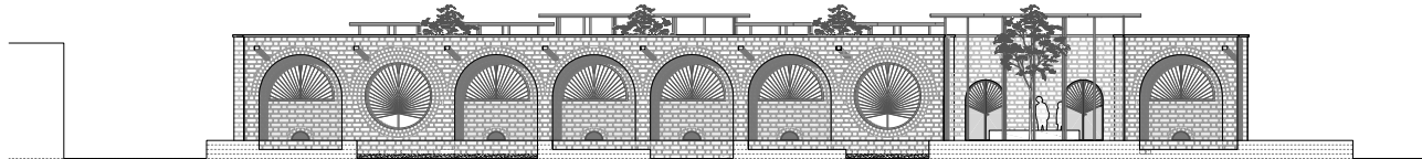
Ansicht | Élévation
