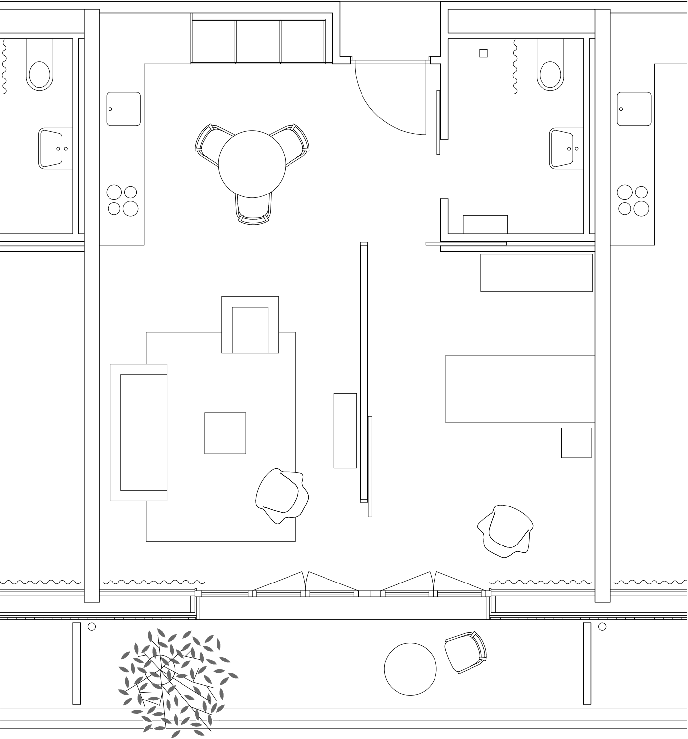
Appartement 2 pièces 1:50
