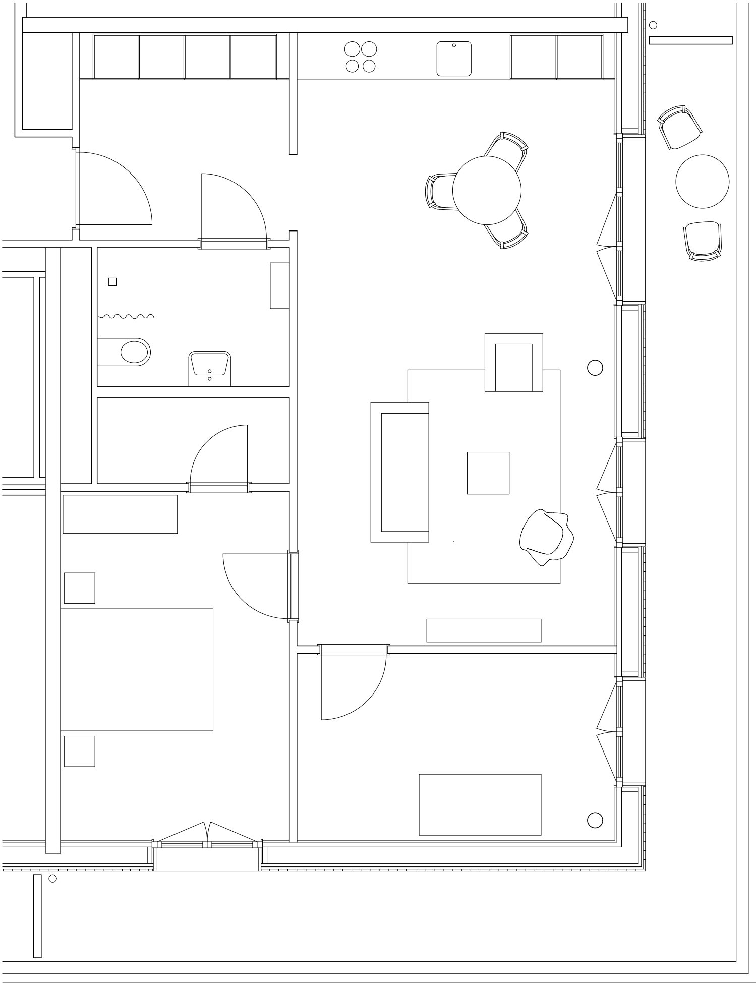
Appartement 3 pièces 1:50
