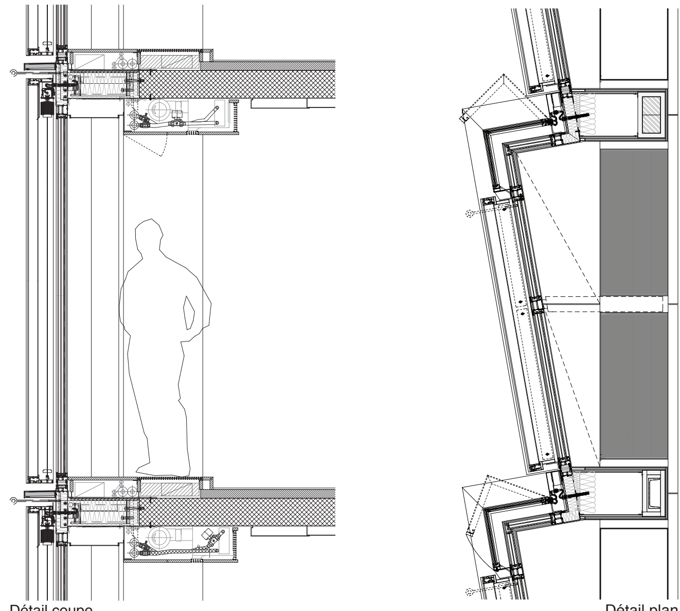
Détail coupe
