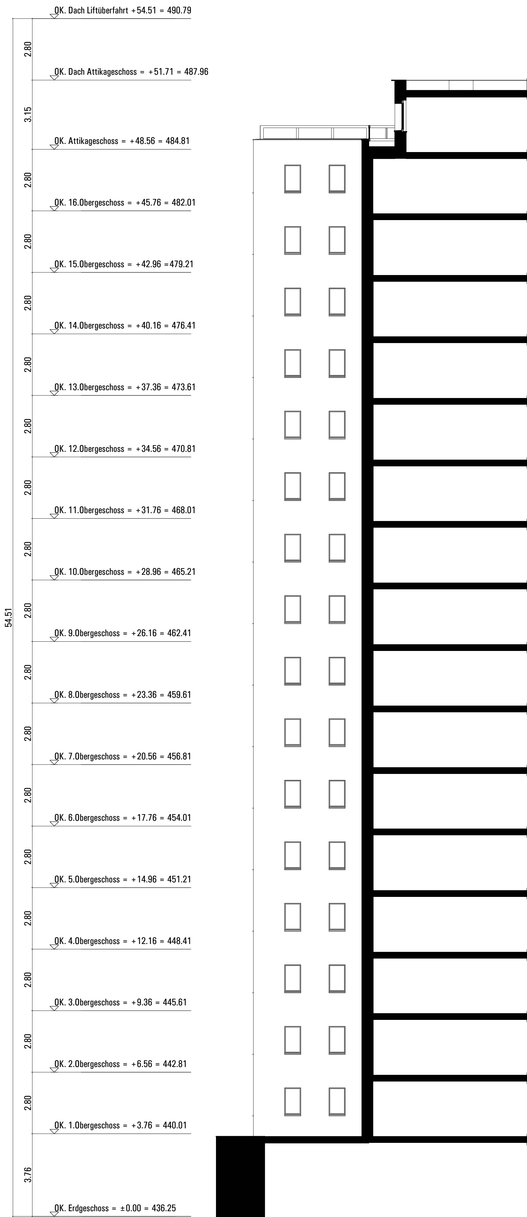
Schnittansicht Richtung Osten
