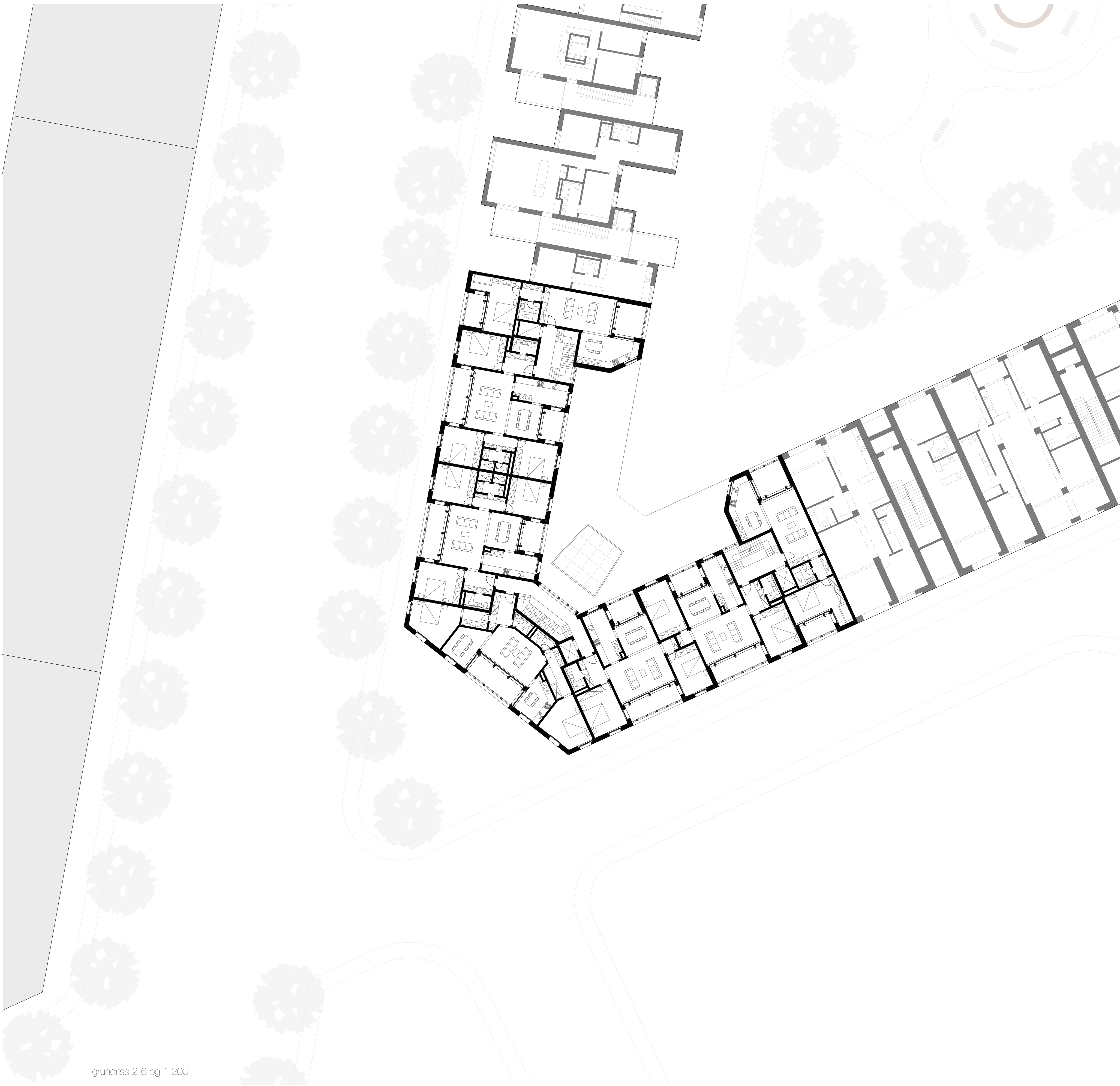
grundriss 2-6 og 1:200
