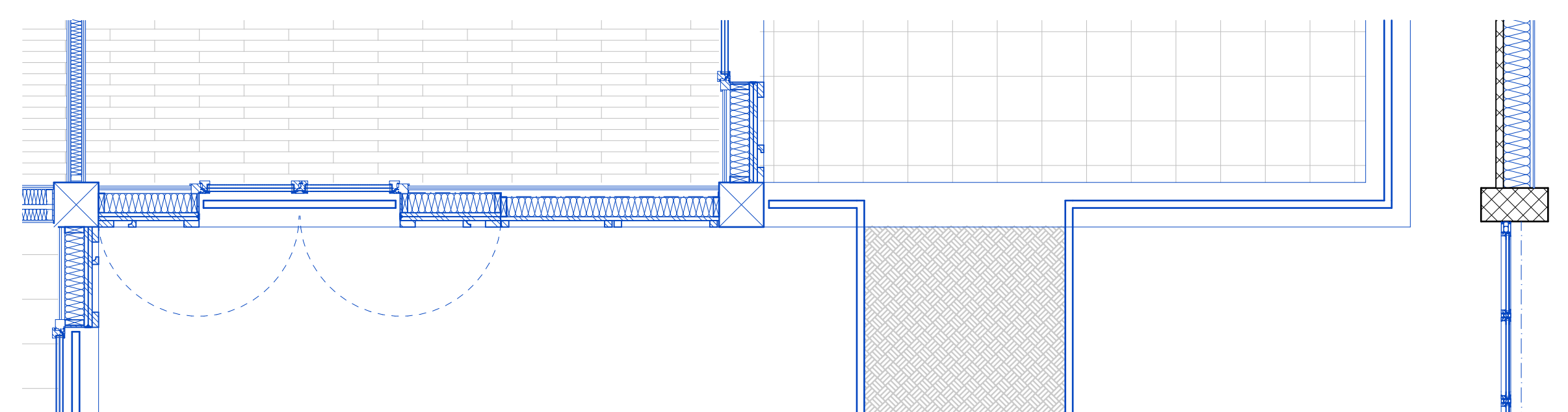
Detailgrundriss 1.Obergeschoss | 1:33
