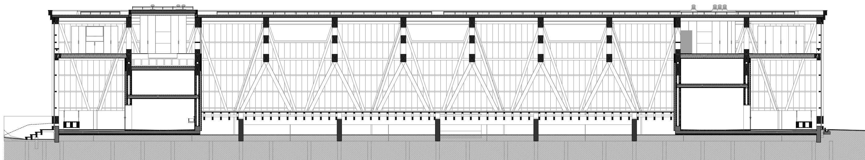
Schnitt F-F
