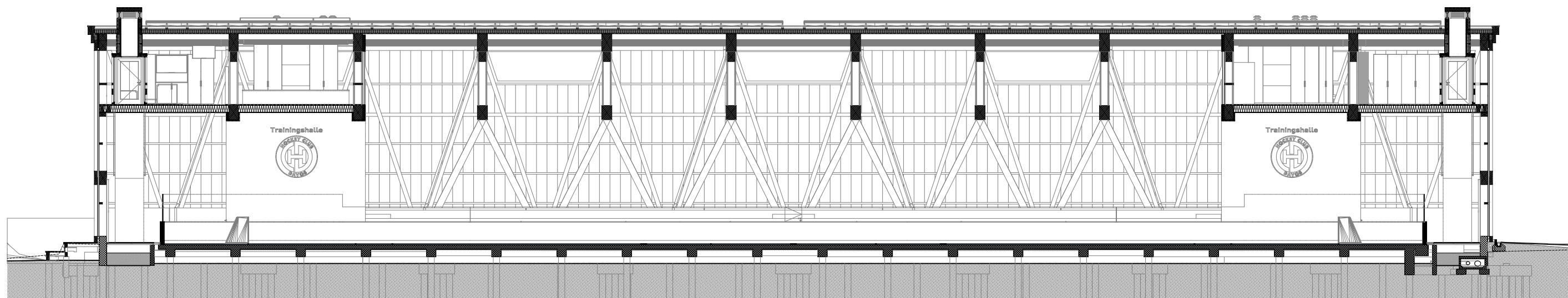
Schnitt H-H
