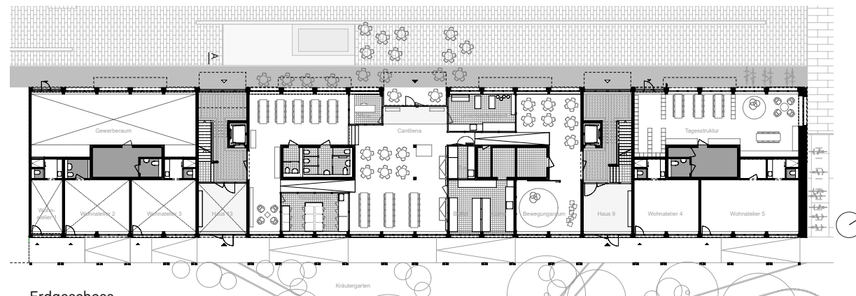
Erdgeschoss Rez-de-chaussée
