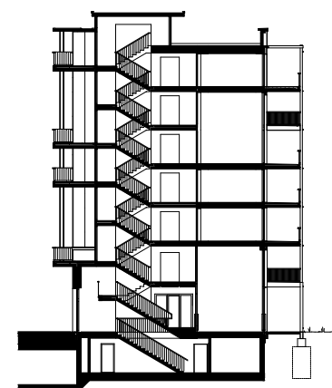
Schnitt A Coupe A
