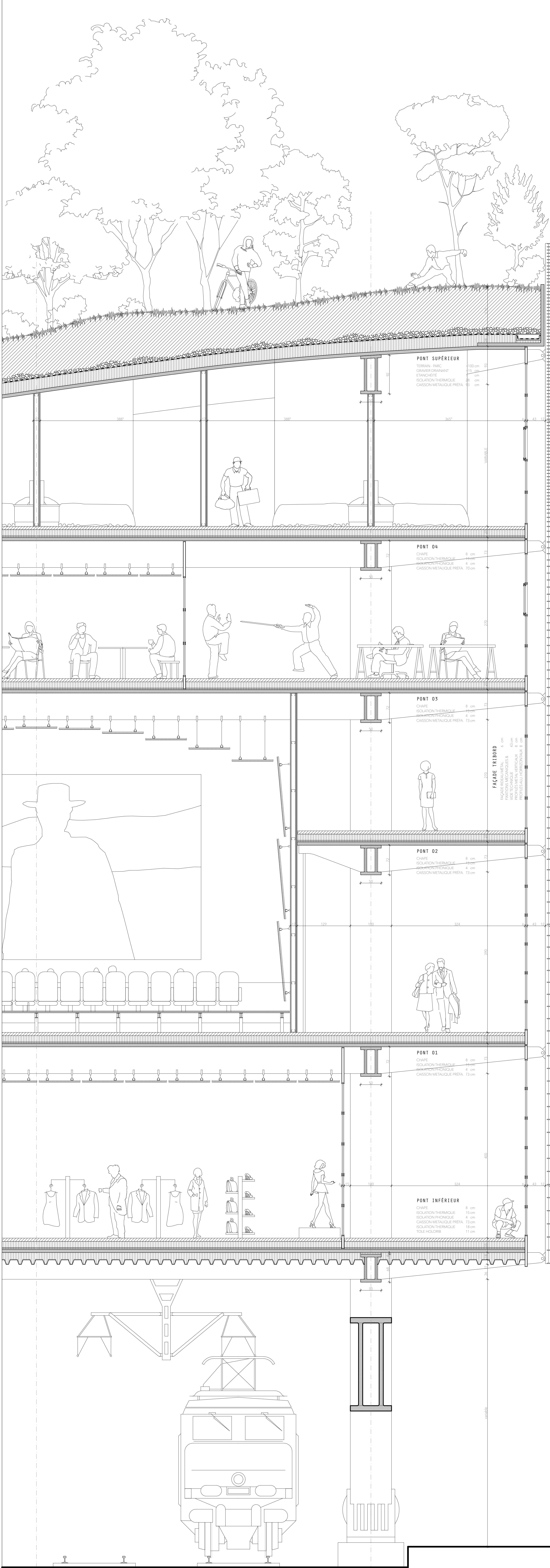
DÉTAIL CONSTRUCTIF / EXTRAIT DE FAÇADE
