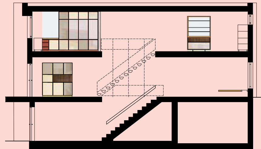
Schnitt B | Coupe B
